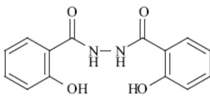
Salicylhydrazide
