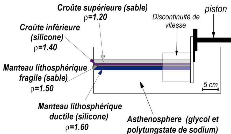
Figure III.3.1. : Dispositif expérimental (vu de côté)
