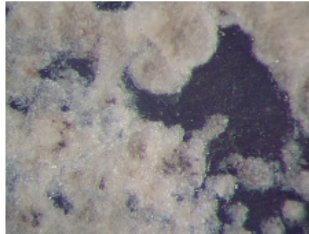
Photo V1e : fragment de vitrail du XIII ème siècle, détail de la corrosion, face externe. 13,5×
