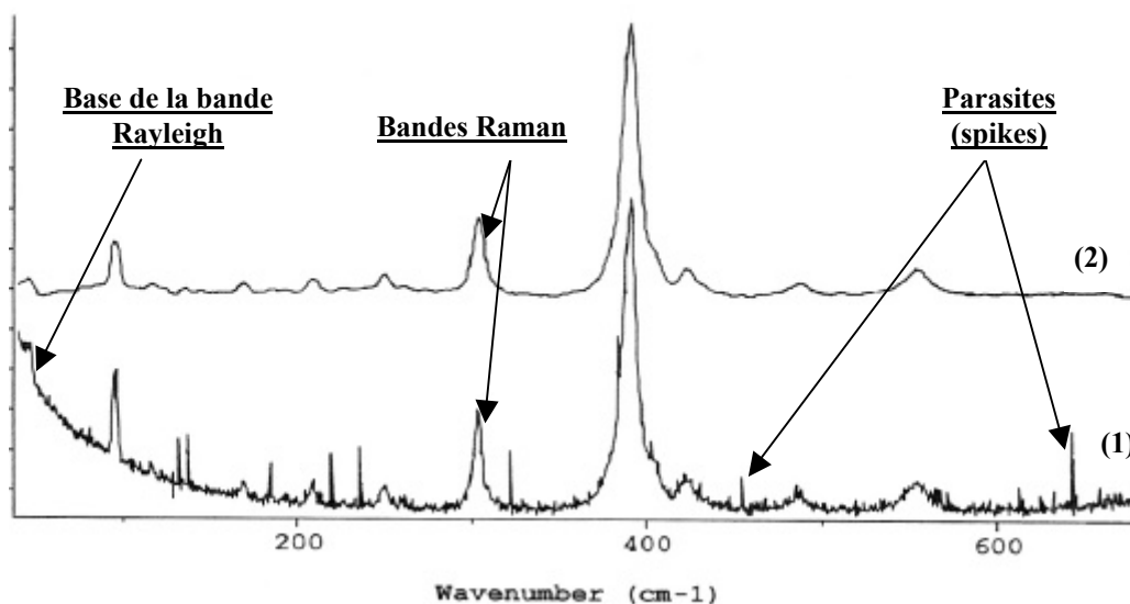
Spectre(s) Raman {1} d'une goethite. (1) brut, (2) après traitement informatique adapté.
