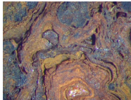
Photo G5 : détail agrandi d'un type de corrosion sur le lingot en fer (L1) ; grossissement : 8,3×
