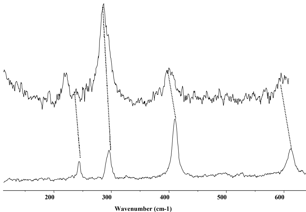
Spectre(s) Raman {37} d'une hématisation archéologique chauffée (clou P.547 ) (spectre du haut) - BYFE16- et hématisation étalon (spectre du bas), Fiche 3 - ACHT14-
