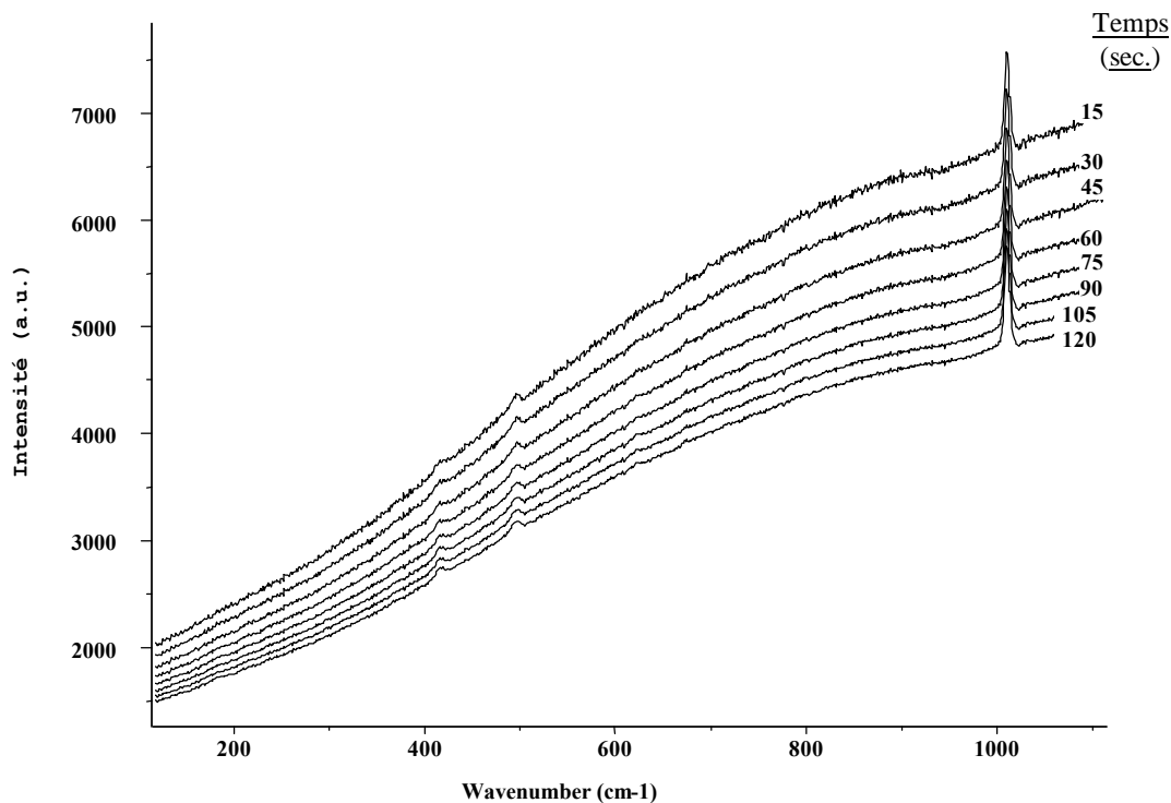
Spectre(s) Raman {2} du gypse identifié sur un vitrail du XVII-XVIII ème siècle. La fluorescence peut être réduite par une prolongation de l'exposition (temps en sec.) de l'échantillon sous le laser -de haut en bas, DGVI 3 à 10-
