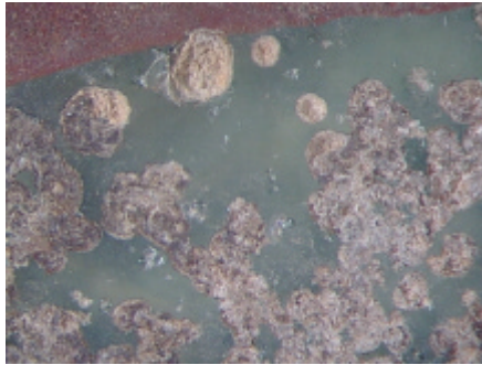
Photo V1d : fragment de vitrail du XIII ème siècle, détail de la corrosion, face interne. ~8×
