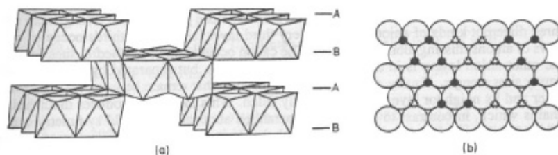
Figure 15. Structure de la goéthite ; (a) présentation en couches d'octaèdres, (b) distribution pour une couche d'anions ; les petits cercles représentent les cations selon leur position par rapport à la couche d'anions; selon Waychunas, 1991.
