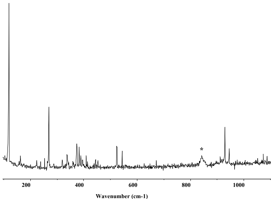
Spectre(s) Raman {3} des raies plasma du laser vert à ions Ar + (acquisition sans filtre interférentiel). Les bandes marquées d'un astérisque correspondent aux bandes de l'objectif du microscope (voir ci-dessous).
