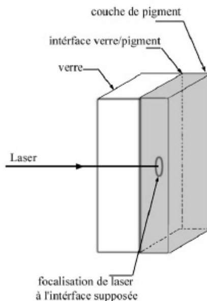
Figure 42. Mode d'analyse par MR, en transparence, de l'interface pigment/verre.
