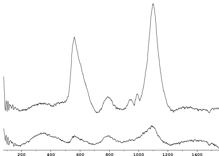
Spectre(s) Raman {48} du verre cordelé .
