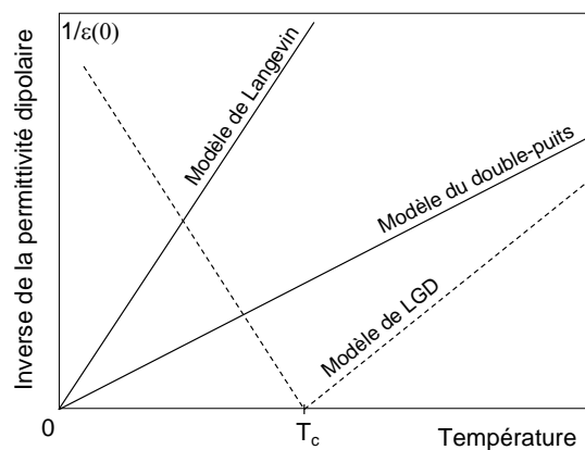
FIG. 1.16 – Caractéristiques 1/\varepsilon(0) en fonction de la température selon les trois modèles de polarisation dipolaire.
