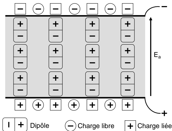
FIG. 1.6 – Représentation schématique de la polarisation dans un diélectrique. E_a désigne le champ électrique appliqué aux bornes du condensateur.
