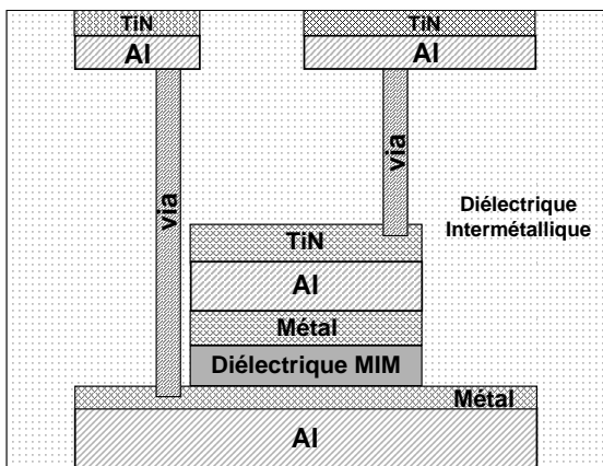
FIG. 8 – Capacité MIM planaire dans un BEOL aluminium.
