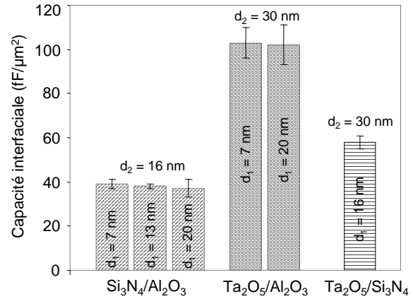
FIG. 4.34 – Capacités interfaciales des différents empilements diélectriques : d_1 est l'épaisseur de la couche inférieure, d_2 celle de la couche supérieure.
