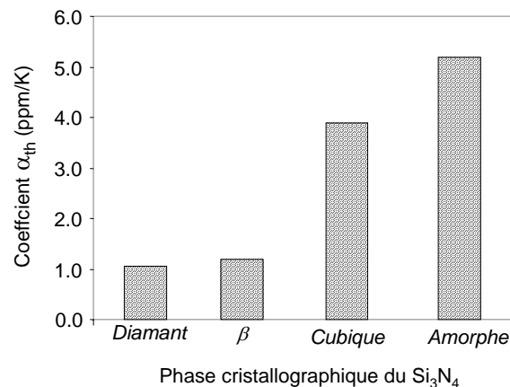
FIG. 4.26 – Coefficient linéaire de dilatation thermique du nitrure de silicium en fonction de sa phase cristallographique. Les données de la phase amorphe sont issues de notre étude.
