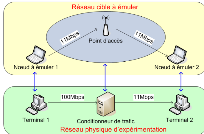
FIG. 3.3: Exemple d'utilisation d'un conditionneur de trafic
