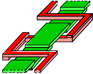
Figure 45 : Micro-bobines intégrées sur silicium.
