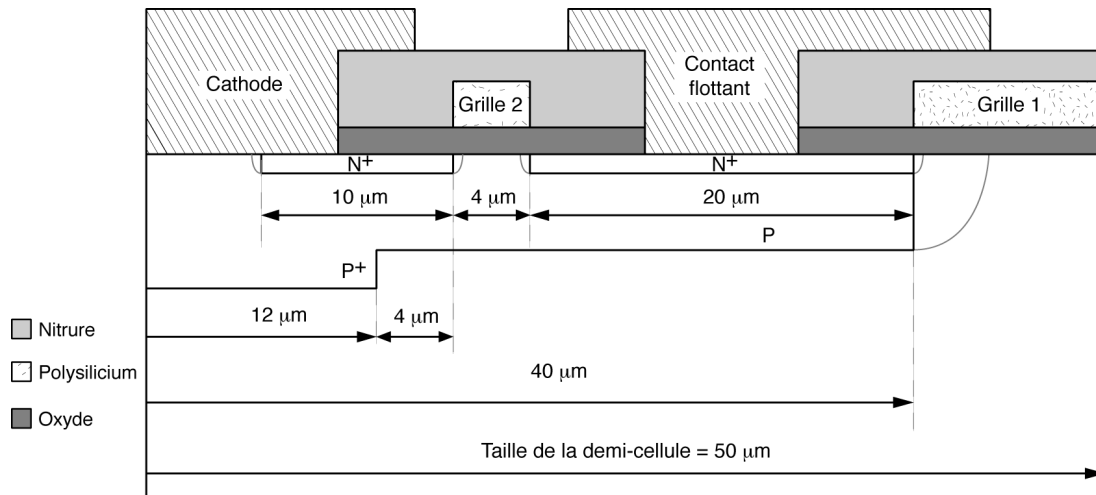
Figure 26 : Règles de dimensions pour la demi-cellule EST.
