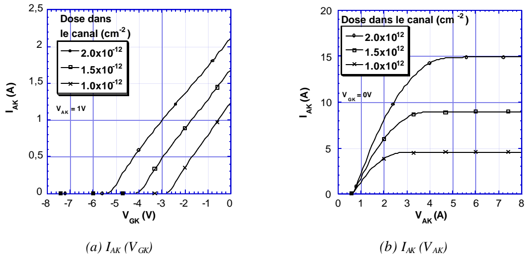
Figure 21 : Caractéristiques électriques statiques d'un IGBT à canal préformé [1].
