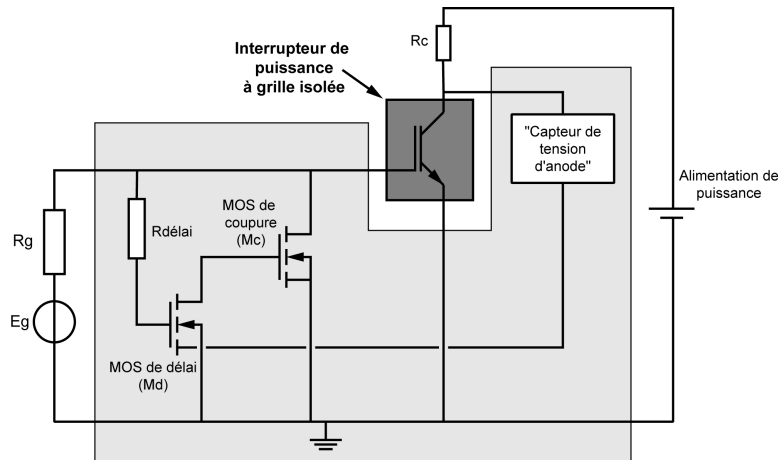
Figure 43 : Schéma de principe du circuit de détection et de protection contre les courts-circuits [55].
