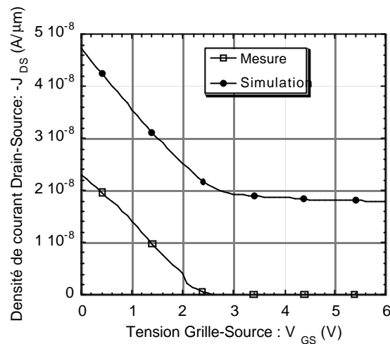
Figure 40 : Comparaison de la caractéristique -J_{DS}(V_{DS}) entre simulation et mesure ; E=120 keV, D=2.10^{12} cm ^{-2} .
