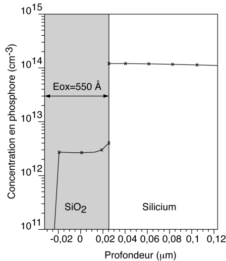
Figure 3 : Epaisseur d'oxyde de grille (simulation 1D).
