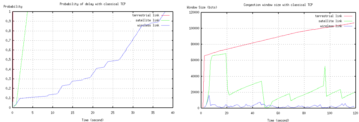
Figure II-6 - Comportement d'une souche TCP sur des réseaux Hertziens
