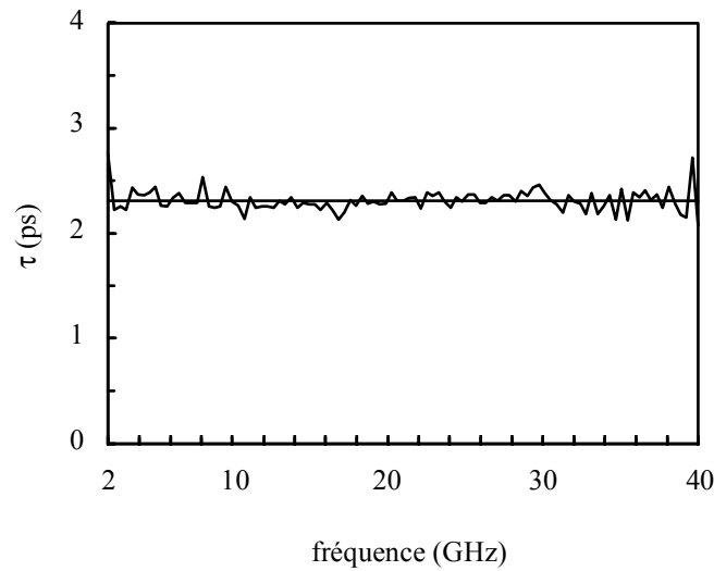
Figure 15 : Variations du temps de transit d'un TBH GaInP/GaAs en fonction de la fréquence
