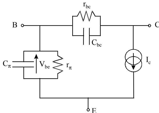
Figure 12 : Schéma électrique intrinsèque en \Pi d'un TBH
