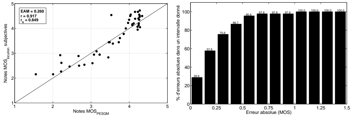
(a) Mapping entre notes moyennes de locution subjectives et objectives (PESQM) (b) Distribution cumulative de l'erreur absolue entre notes moyennes de locution subjectives et objectives (PESQM)
