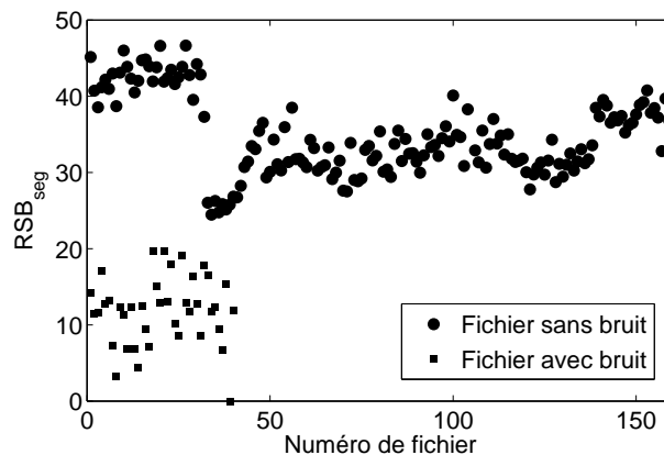
Figure 5.4 : Calcul du rapport signal-à-bruit segmental sur les fichiers (sans ou avec bruit) de la base d'apprentissage
