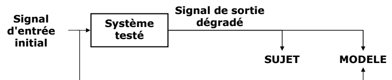
(a) Le sujet juge le signal dégradé, en comparaison avec sa référence de qualité interne
