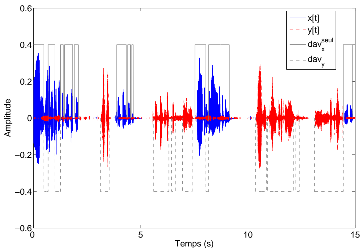
Figure 4.12 : Exemples d'application de l'algorithme de découpage des signaux à des signaux de conversation enregistrés durant le test 1
