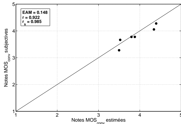
Figure 3.24 : Mapping entre notes de conversation subjectives et estimées - Conformité avec le test 1 pour les conditions avec délai et écho - Test 4 sur l'écho, le délai et les pertes de paquets
