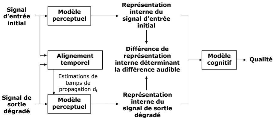
(b) Le modèle PESQ transforme le signal dégradé et le signal de référence correspondant en représentations internes, puis utilise leur différence pour calculer une note de qualité d'écoute
