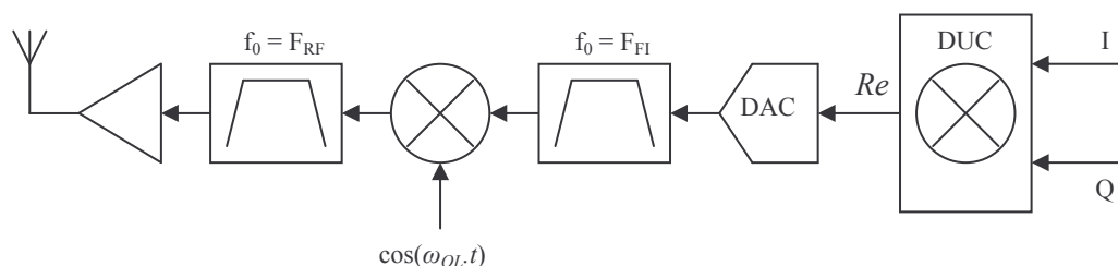
figure 92 : Architecture d'émission à FI numérique
