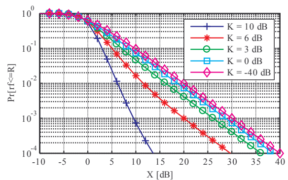
figure 7 : Probabilité que l'enveloppe du signal soit inférieure à R en canal de Rice
