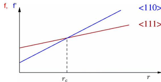
FIG. 5.16 : Représentation schématique de l'énergie libre par unité de longueur f ( \mathbf{f}=\mathbf{F}/\mathbf{L} ) en fonction du rayon des nanofils orientés selon \langle 111 \rangle et \langle 110 \rangle après croissance sur un substrat de Si(001) [30].
