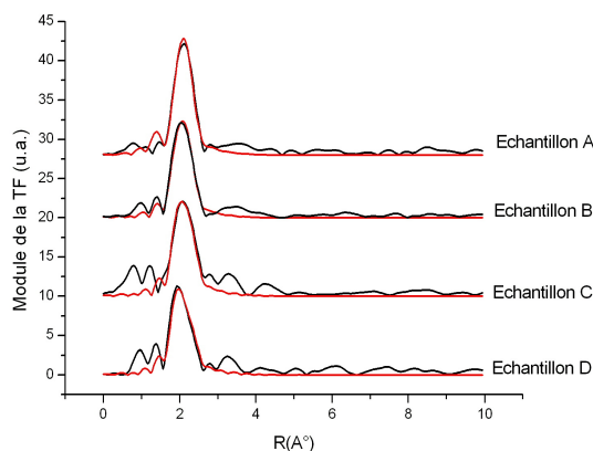
FIG. 3.12 : Transformée de Fourier des oscillations \chi(k) multipliées par k^3 pour les différents échantillons étudiés. Les spectres expérimentaux sont représentés en noir tandis que les courbes d'ajustement apparaissent en rouge.
