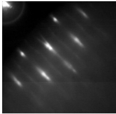
FIG. 1.13 : Image RHEED dans la direction [100] d'un dépôt de 4 MC de Ge à 550\text{ }^{\circ}\text{C} . Les tiges de diffraction ou "strikes" proviennent des facettes \{105\} présentes sur les îlots huttes.
