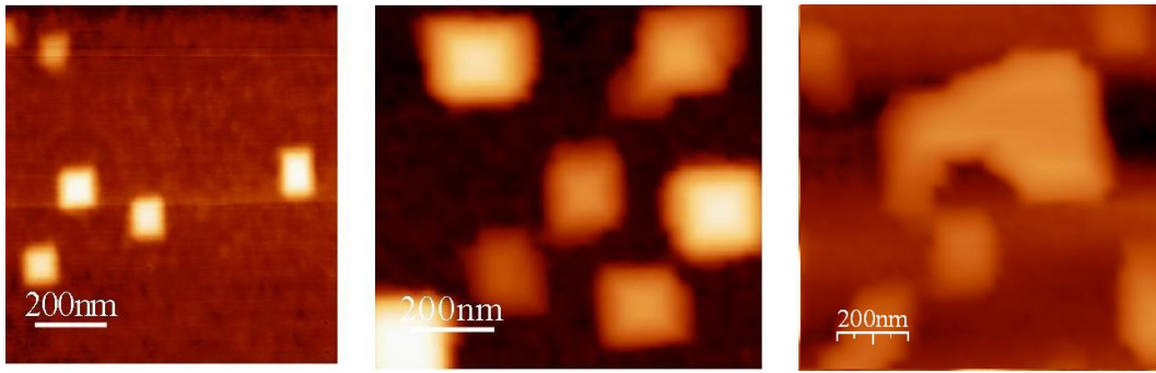
FIG. 4.6 : Images AFM d'îlots de Si épitaxiés à travers SiO 2 avec (a) 1,2 nm (épaisseur équivalente) de Si déposé, (b) 3,5 nm et (c) 4,5 nm.
