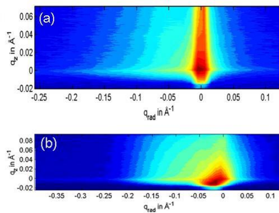
FIG. 3.8 : Cartographie de diffraction des rayons X réalisée suivant la direction radiale dans le plan autour du pic de Bragg (220) du Si pour : (a) des boîtes de Ge épitaxiées à travers \text{SiO}_x (échantillon A) et (b) des boîtes de Ge épitaxiées à travers \text{SiO}_2 (échantillon C). Q_{rad} et Q_z représente respectivement les composantes du moment de transfert dans la direction radiale ( Q_{rad} = \frac{4\pi}{\lambda} \sin \theta ) et dans la direction perpendiculaire au plan.
