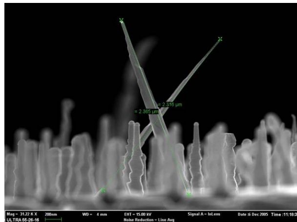
FIG. 5.18 : Image MEB de deux nanofils tiltés par rapport à la direction \langle 111 \rangle . Le diamètre de ce nanofil est de l'ordre de 30 nm vers leur sommet
