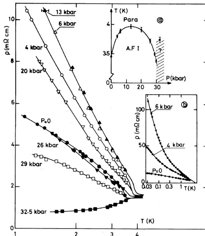
FIG. 3.9 : Résistivité de TmSe sous pression; le premier insert montre le diagramme de phase déduit de ces mesures et le deuxième insert précise des mesures à très basses températures.
