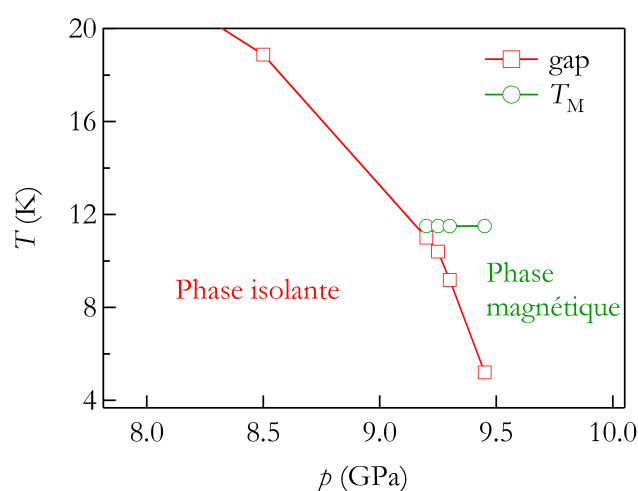
FIG. 4.15 : Diagramme de phase de SmB_6 : zoom aux alentours de la pression critique d'après notre seconde mesure en cellule à enclume diamant. Voir annexe pour le détail des mesures
