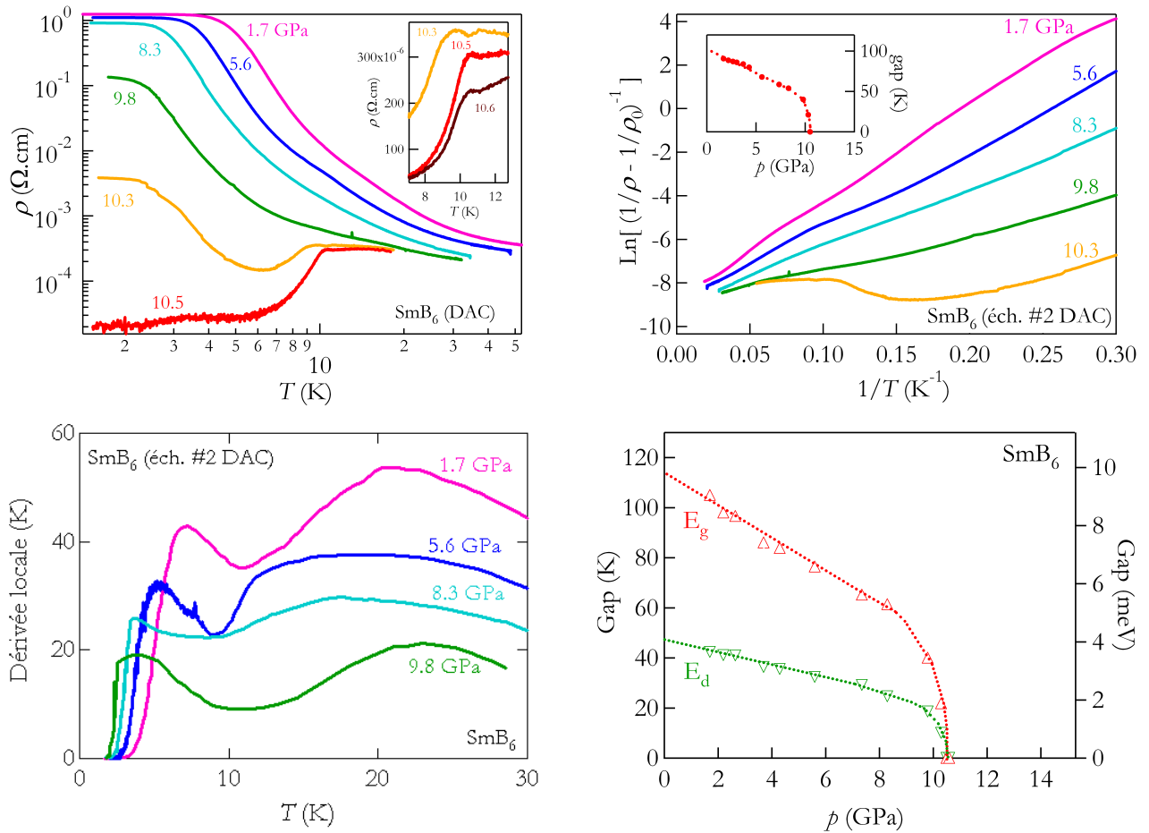
FIG. 4.10 : Résultats obtenus par mesure de résistivité sur l'échantillon 2 dans la cellule à enclume diamant. (a) Données brute de résistivité en fonction de la température pour quelques pressions : 1.7, 5.6, 8.3, 9.8, 10.3 et 10.5 GPa. En insert un zoom a été effectué pour les trois plus hautes pressions mesurées (10.3, 10.5 et 10.6 GPa) au niveau de l'anomalie magnétique ; (b) tracé d'Arrhenius et évolution correspondante du gap dans la phase isolante ; (c) Énergie locale d'activation (dérivée) pour les mêmes pressions qu'en (a) ; (d) Estimation de l'évolution du gap en fonction de la pression déduit de la dérivée locale.
