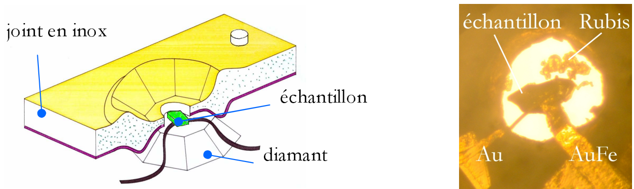
FIG. 2.7 : Zoom au niveau de la chambre de pression. À gauche un dessin schématique (d'après [THOMASSIN, 2000]) du joint de la cellule (l'isolation est représentée en violet), à droite une photo de l'échantillon installé dans la chambre de pression
