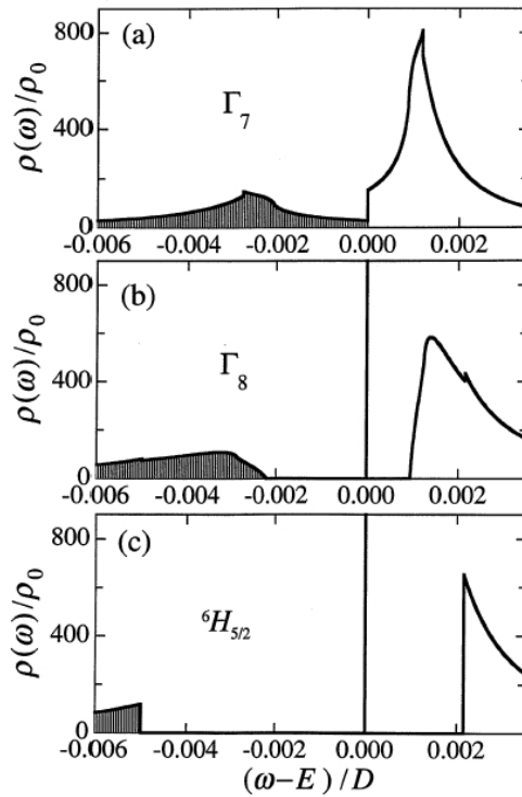
FIG. 1.14 : Densité d'état fermionique en fonction de l'énergie pour trois cas limites : (a) \Gamma_7 , (b) \Gamma_8 et (c) {}^6H_{5/2}
