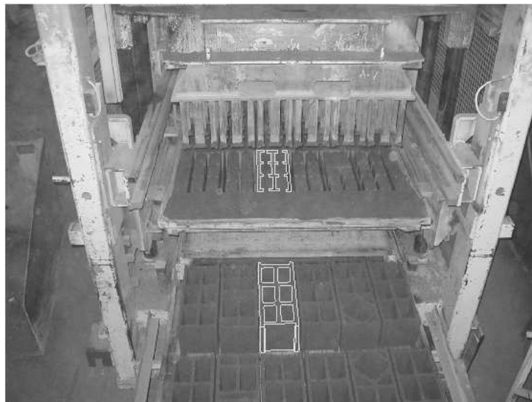
Figure 1.12 – Photo d'une presse vibrante lors de la sortie des produits
