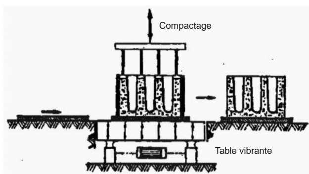
Figure 1.6 – Machine fixe européenne pour la production de blocs
