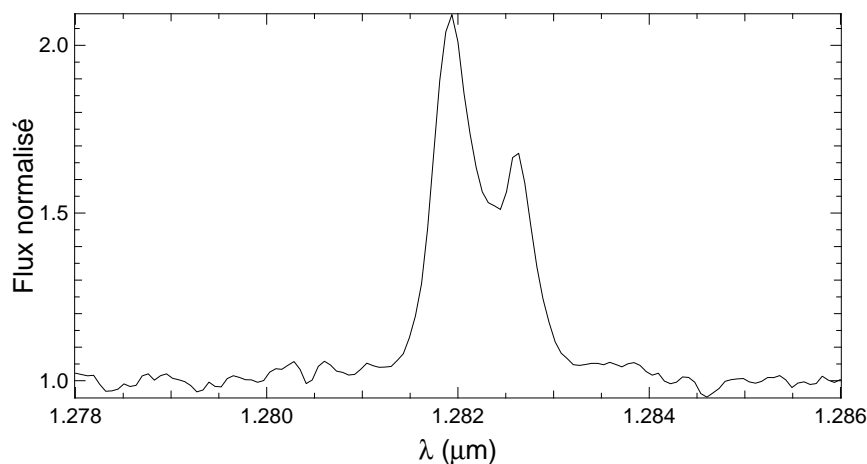
FIG. 6.3 — Profil de la raie Pa. \beta de l'étoile \kappa CMa, montrant un dédoublement caractéristique, associé dans ce cas à un disque en rotation, ainsi qu'une asymétrie, interprétable comme une inhomogénéité de ce disque.
