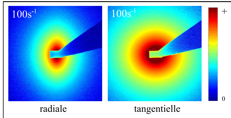
Fig. 11.3 Images en position radiale et position tangentielle de SAXS de la solution PEO 4% et Sépiolite 0,5% en volume à 100 s^{-1}
