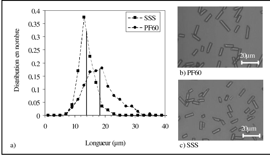
Fig. 11.18 Bâtonnets de verre. a) Distribution de longueur. b) Image microscopique des bâtonnets PF60 de longueur moyenne 18,3 µm. c) Image microscopique des bâtonnets SSS de longueur moyenne 13,8 µm.
