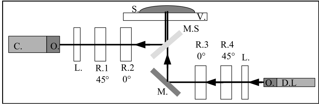
Fig. 5.5 Schéma du dispositif expérimental avec D.L. : Diode Laser ; O. : Optique ; L. : Polariseur linéaire ; R. : Retardeur à cristaux liquides ; M. : Miroir ; M.S. : Miroir semi-transparent, C. : Caméra CCD, V. Vitre et S. Échantillon
