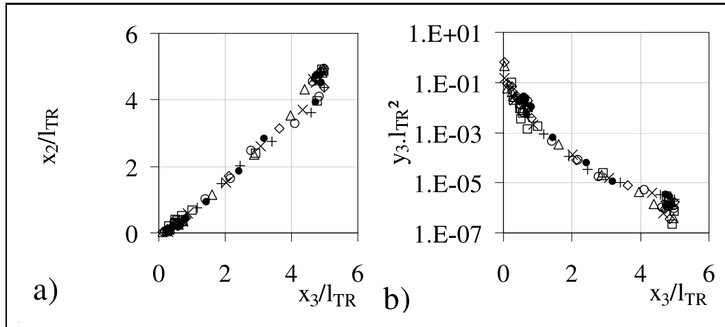
Fig. 7.9 Corrélations entre les informations contenues dans l'élément M_{44} . (+ m = 0,75 , \circ m = 0,90 , \bullet m = 1,10 , \times m = 1,20 , \triangle m = 1,30 , \diamond m = 1,50 , \square m = 1,80 )
