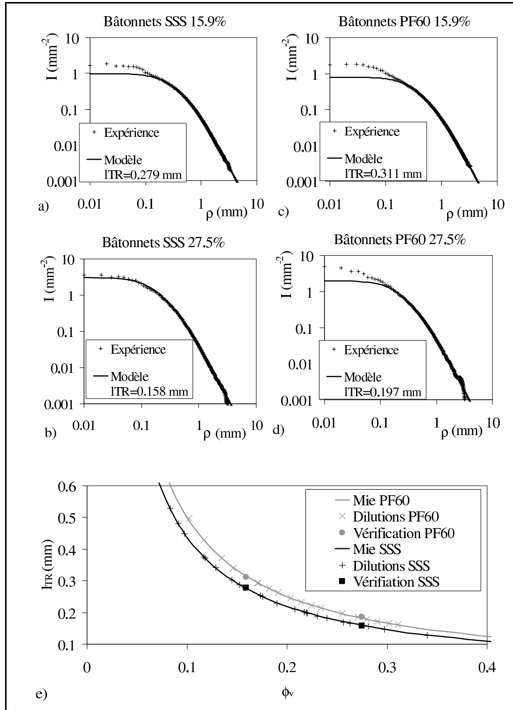
Fig. 11.20 Validation de la mesure de la fraction volumique par inversion de Mie. Ajustement des décroissances radiales d'intensité pour les deux points de vérification pour les bâtonnets SSS (a) et (b) et pour les bâtonnets PF60 (c) et (d). e) Validation, les courbes de Mie sont calculées avec le paramètre optique m = 1,114 et un rayon de particule de 4,51 \mu m pour les bâtonnets SSS et de 4,98 \mu m pour les bâtonnets PF60
