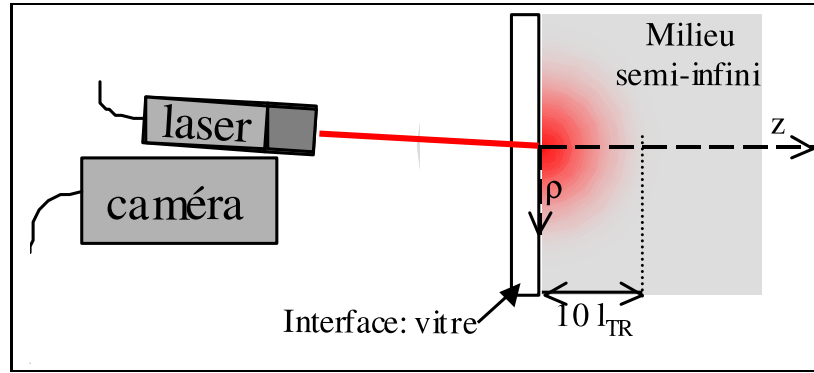
Fig. 4.3 Schéma de rétrodiffusion
