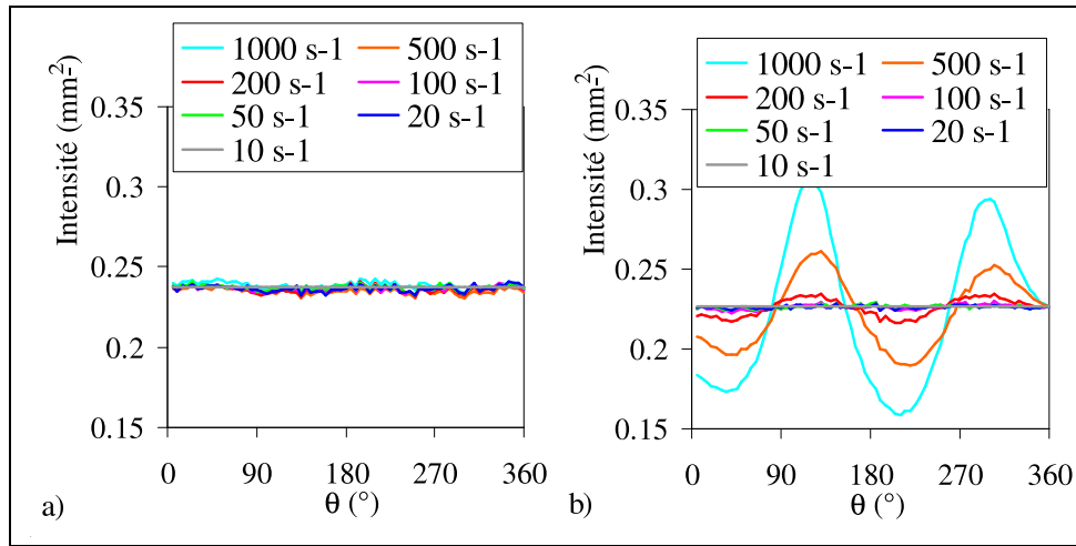
Fig. 12.9 Variations angulaires d'intensité 10 \text{ s}^{-1} à 1\,000 \text{ s}^{-1} pour l'échantillon de disques durcis (a) et de disques déformables (b).
