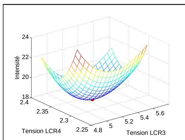
Fig. 5.16 Détection : Optimum générateur de l'état VI. Le point rouge correspond au minimum d'intensité V_{LCR3} = 5,30 \text{ V} et V_{LCR4} = 2,34 \text{ V}
