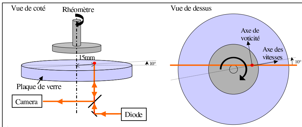
Fig. 5.18 Positionnement du point d'impact laser sur la g om trie du rh om tre
