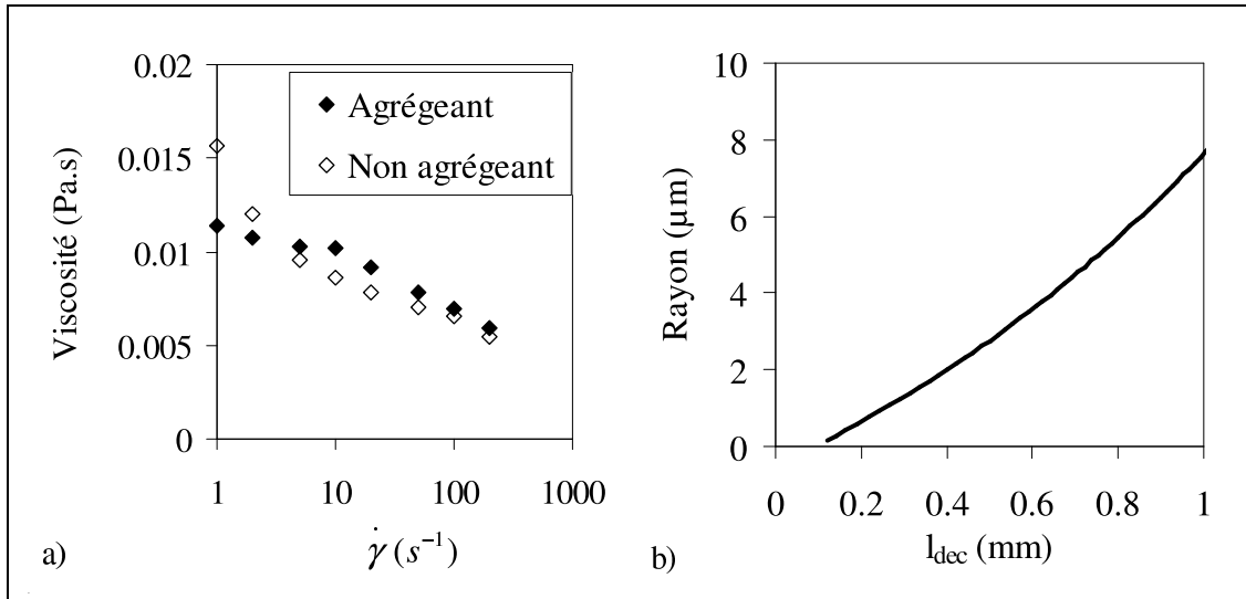
Fig. 12.4 a) Viscosités du sang agrégant et non-agrégant en fonction du cisaillement. b) Inversion de Mie sur l_{\text{dec}} connaissant à la fois les propriétés optiques ( m = 1,045 ) et les fractions volumiques ( \varphi_v = 39\% ).
