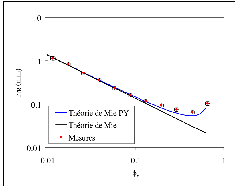
Fig. 4.8 Valiation de l_{TR} pour l'Emulsion2
