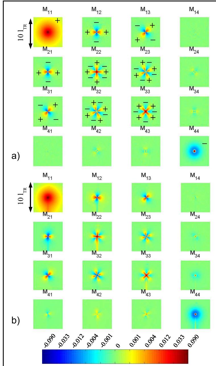
Fig. 8.3 Comparaison des matrices de Mueller en espace et intensité normalisés : a :Simulation de Monte Carlo x = 3 et m = 1 , 1 et b :Expérimentale Emulsion2 (Concentration 1,7%, Rayon moyen 220 nm l_{TR} = 0,80 mm)
