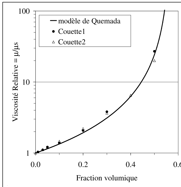
Fig. 2.1 Validation de la modélisation viscosité relative - fraction volumique sur des particules de 300\ \mu\text{m} de diamètre suspendues dans une solution newtonienne de glycérol et d'eau avec \varphi_p = 0.63
