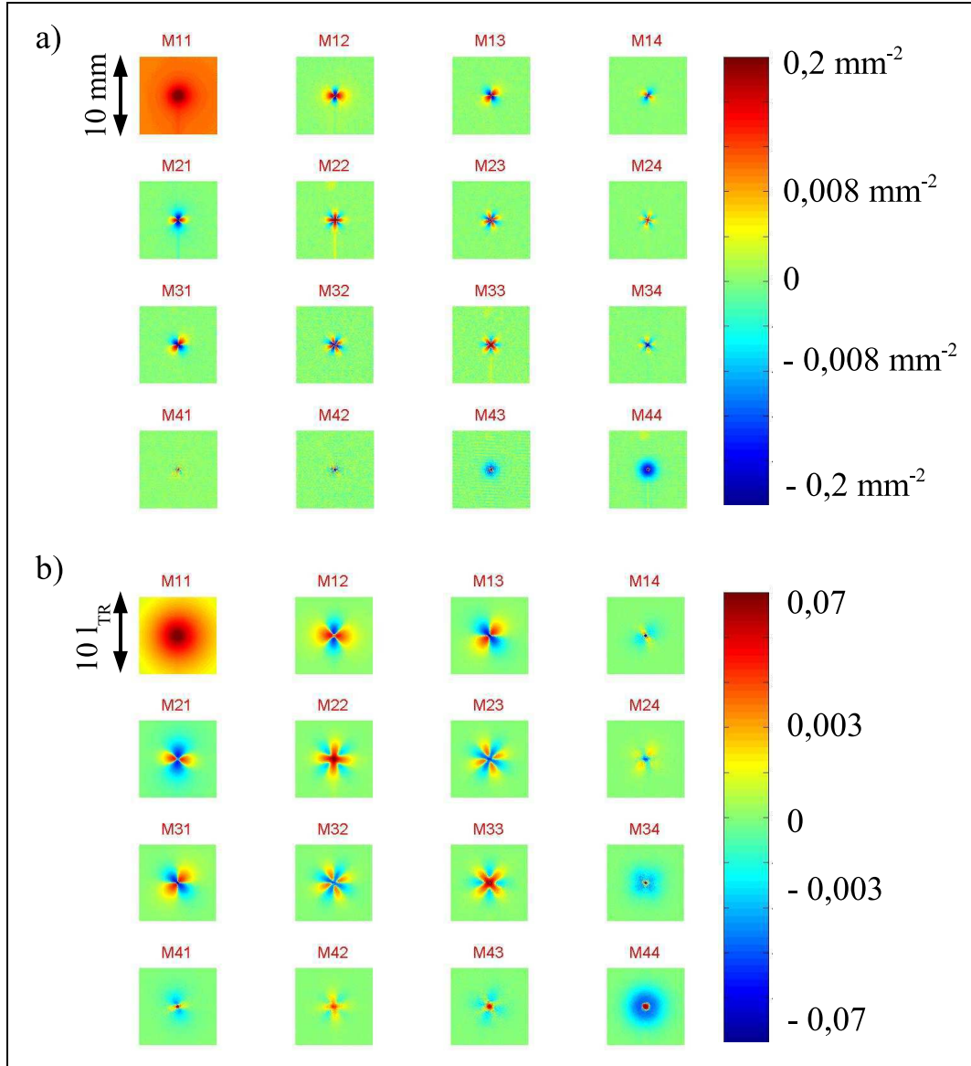
Fig. 5.23 Normalisation d'une matrice de Mueller. Exemple de l'Emulsion2 à une concentration volumique 3,9% avec l_{TR} = 0,34 \text{ mm} . a) Représentation réelle, images de 10 \text{ mm} de coté. b) Représentation normalisée, images de 10 l_{TR} de coté.
