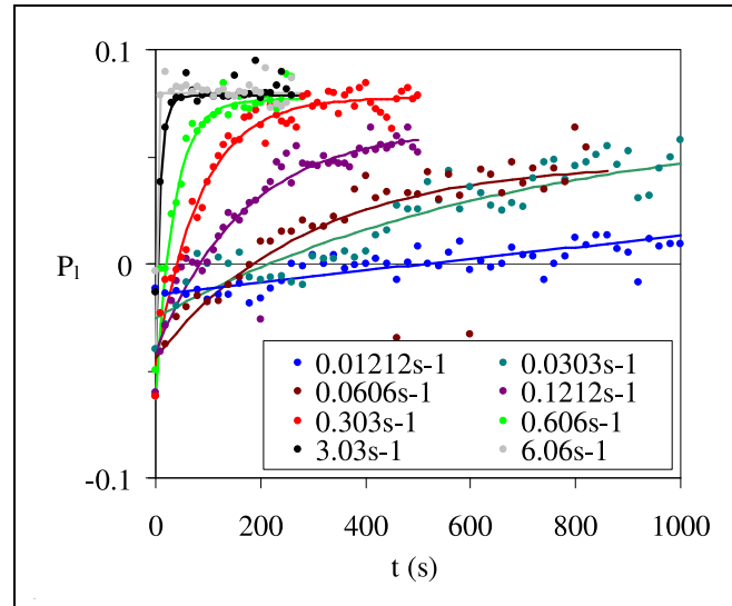
Fig. 11.24 Orientation des bâtonnets PF60 (20,3%) pour différents gradients de vitesse en fonction du temps. Les lignes continues sont les modélisations obtenues avec des corbes exponentielles.
