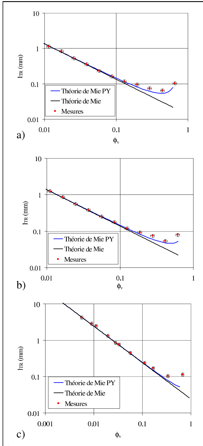
Fig. 8.2 Validation du transport scalaire isotrope de lumière : Comparaison entre la théorie (Mie et Mie Percus-Yevick) et les mesures expérimentales de l_{TR} des émulsions. a : Émulsion 2 avec a[4, 3] = 220 \text{ nm} . b : Émulsion 4 avec a[4, 3] = 375 \text{ nm} . c : Émulsion 5 avec a[4, 3] = 970 \text{ nm} .
