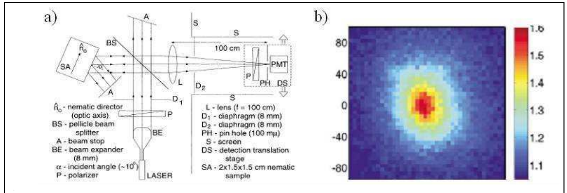
Fig. 2.2 a. Dispositif de mesure du cône cohérent de lumière, (Vithana et al., 1993). b. Image 2D anisotrope d'un cône cohérent de lumière obtenue sur des cristaux liquides orientés, (Sapienza et al., 2003).
