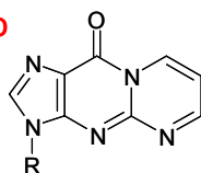
M 1 -dGuo
