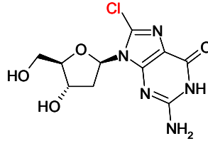
8-Chloro-2'-désoxyGuanosine (8-ClGuo)
