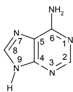
Adénine
