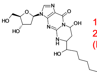
1,N 6 -éthéno-2' désoxyadénosine (εdAdo)
