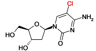
5-Chloro-2'-désoxyCytidine (5-ClCyd)
