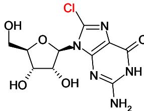
8-ChloroGuanosine (8-ClGuo)
