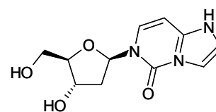
3,N 4 -éthéno-2' désoxycytidine (εdCyd)
