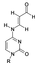
M1-dCyd
