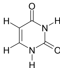
Figure 13 : Structure chimique de l'uracile.
