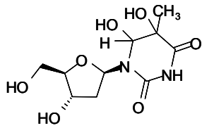
Diols de thymidine (Gly-Thd)
