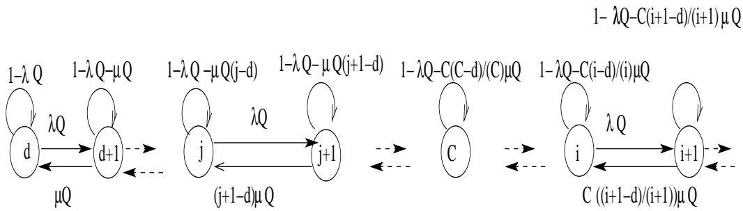
FIG. 4.3: Chaîne de Markov lorsque d < C
