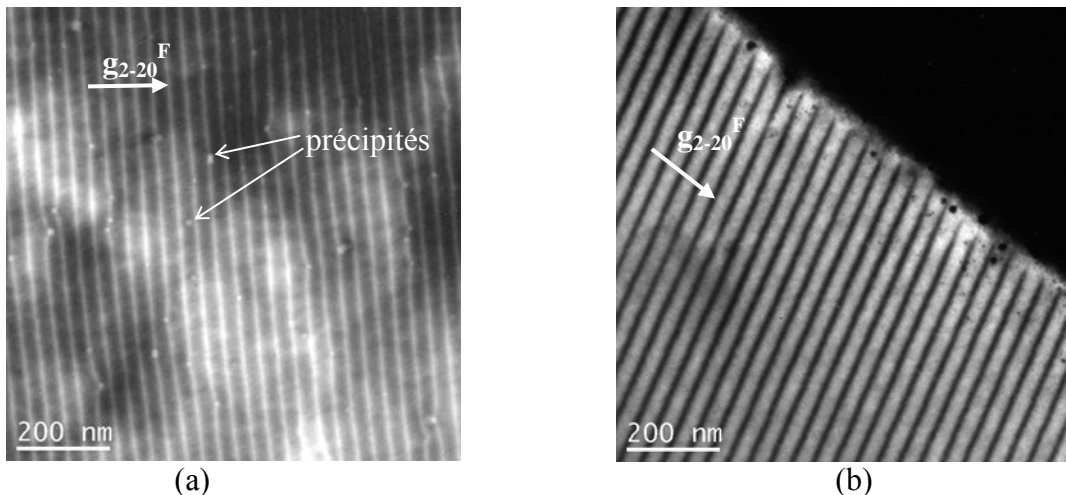
Figure 65 : Clichés MET en vue plane, mode deux ondes en champ sombre. (a) substrat C3 (recuit T=1100°C) : on observe la présence de précipités de SiO 2 . (b) substrat C1 (recuit T>1100°C) : absence totale de précipités de SiO 2 .
