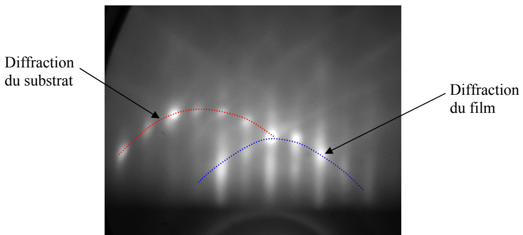
Figure 69 : Cliché RHEED obtenue avec un échantillon de la plaque C4 (C4-1), après un traitement thermique à 800^\circ\text{C} . On observe la reconstruction 2 \times 1 du Si désoxydé. L'image est prise dans l'azimut [110] du film, le diagramme de diffraction du substrat (en rouge) est décalé de 2,2^\circ .
