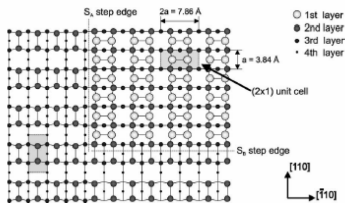
Figure 5 : Schéma de la reconstruction (2×1) de la surface (001) du silicium avec terrasses. La terrasse supérieure (en haut à droite) est séparée de la marche inférieure (à gauche) par les limites S_A et S_B . Une cellule rectangle unitaire est représentée en gris sur chacune des terrasses. A cause de la symétrie diamant du silicium, cette cellule est tournée de 90^\circ entre les deux terrasses.
