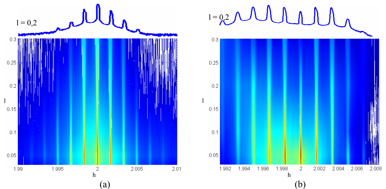
Figure 86 : Cartographie de l'espace réciproque autour du pic de Bragg (221) du film avec 0,03 \leq l \leq 0,1 , pour (a) un échantillon de la plaque C2 après désoxydation thermique sous flux, et (b) pour l'échantillon C2-3 (dépôt de 6MC de Ge).
