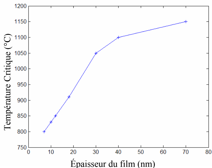
Figure 71 : Courbe expérimentale de la température critique de stabilité du joint de grains pour la plaque C3 ( 20^\circ de torsion et 0,44^\circ de flexion).
