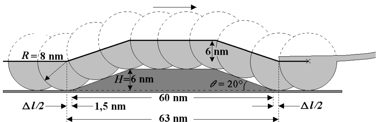
Figure 24 : Profil AFM (trait noir) auquel on remonte en balayant avec une pointe de 8 nm de rayon de courbure un îlot de 6 \times 60 nm (d'angle de contact \theta = 20^\circ ) ; la dimension latérale est surestimée de 5\% ( + 3 nm ici), la hauteur mesurée est elle en revanche fidèle (îlot sans voisin accolé).
