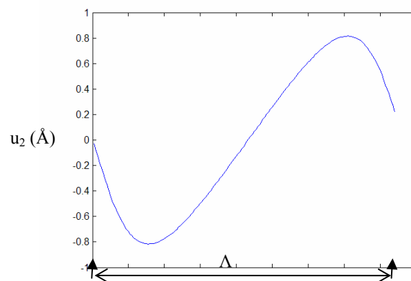
Figure 79 : Simulations du champ de déplacement, hors du plan, à la surface du film, obtenu dans les mêmes conditions que pour les résultats de la figure précédente. Les flèches noires indiquent la position des dislocations.
