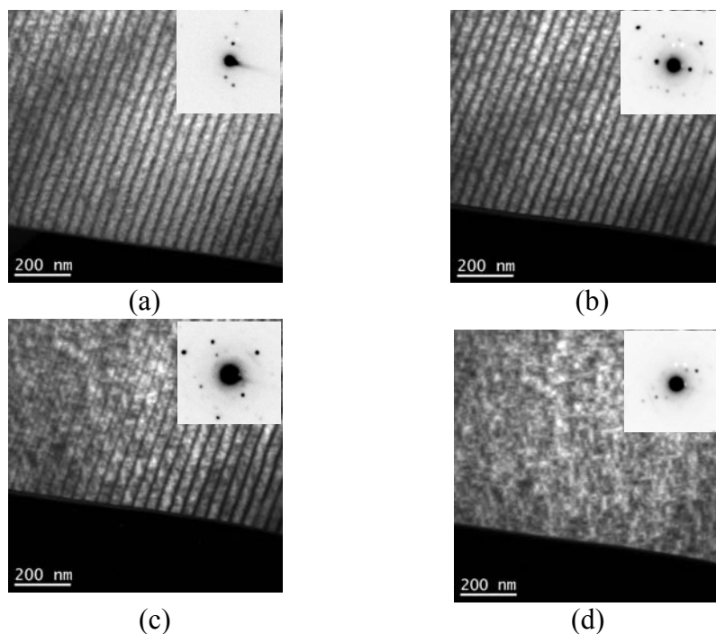
Figure 62 : Images MET en conditions deux ondes approchées, en champ sombre, du substrats C2, en excitant différents g du film. (a) g = (\bar{2}20) , (b) g = (220) , (c) g = (400) , (d) g = (040) . En insert, les clichés de diffraction associés.
