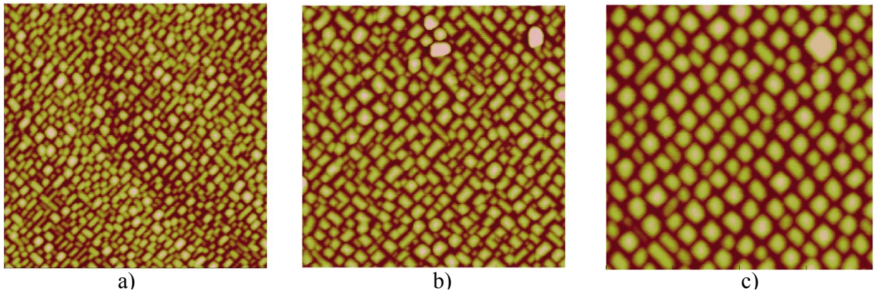
Figure 11 : Image AFM 1\mu\text{m} \times 1\mu\text{m} d'îlots de SiGe sur Si (001) : a) après une seule couche d'îlots, b) après la 2 ème couche d'îlots, c) après la 20 ème couche d'îlots. La dispersion en taille diminue avec le nombre de multicouches SiGe/Si, de même qu'il apparaît une organisation latérale des îlots [35].
