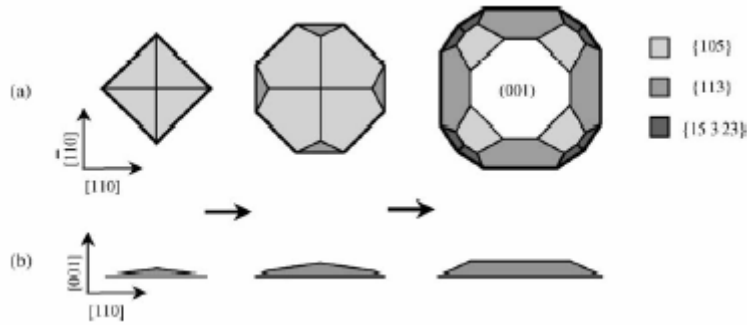
Figure 7 : Illustration de la transition de forme des îlots facettés durant la croissance EJM d'alliage Si_{1-x}Ge_x (avec 0,2 < x < 0,6 ) sur Si(001) avec augmentation de la contrainte (de gauche à droite) : (a) vue de dessus et (b) vue en coupe suivant la direction [110] . Au début, les îlots ont une forme pyramidale présentant des facettes \{105\} . Avec l'augmentation de la contrainte, en plus de ces facettes \{105\} , des facettes plus raides telles que des facettes \{113\} et des paires de \{15\ 3\ 23\} apparaissent, permettant ainsi aux îlots de croître en hauteur. Ces îlots « multi-facettés » ont une forme polygonale et sont couramment appelés « dômes ». En raison de la formation de terrasse (001) au sommet des îlots, ces derniers restent assez plats comme on peut le voir en coupe.
