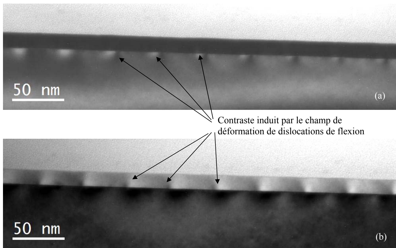
Figure 60 : Image MET en coupe de la plaque C3, dans l'axe de zone [110] (a) du film et (b) du substrat.
