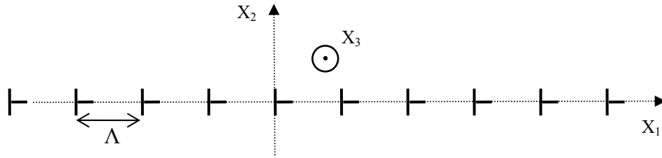
Figure 43 : Choix du repère de coordonnées. Sur ce schéma le vecteur de Burgers de chaque dislocation est \mathbf{b} = b \cdot \mathbf{x}_2 . Remarque : ici le système de coordonnées est tourné de 90^\circ autour de l'axe X_2 par rapport à la figure donnée dans le Hirth et Lothe, pour avoir les même notation tout au long du chapitre : x \rightarrow X_2 , y \rightarrow -X_1
