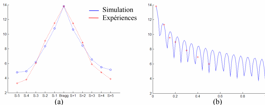
Figure 77 : Comparaison des résultats expérimentaux de diffraction de RX (en rouge) avec les résultats de simulation (en bleu) pour \mathbf{b} = (a_{Si} / 2) \cdot \mathbf{x}_2 . (a) Intensité des pics satellites autour du pic de Bragg (220) du film de la plaque C2. (b) Décroissance du même pic de Bragg en fonction de l'indice l ; les oscillations observées sur cette simulation sont liées à la troncature abrupte suivant l'épaisseur du film.
