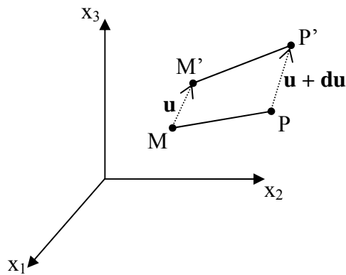
Figure 38 : Les deux points M et P sont proches de manière que MP = dx . Après action d'une contrainte, M et P se déplacent en M' et P' . En notant u le champ de déplacement, u(M) = MM' et u(P) = PP' , et M'P' = dx + du .
