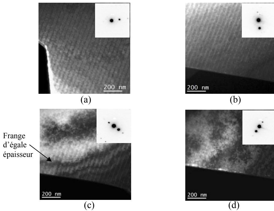
Figure 61 : Images MET en conditions deux ondes approchées, en champ sombre, de la plaque C2, en excitant différents g du substrat. (a) g = (400) , (b) g = (0\bar{4}0) , (c) g = (2\bar{2}0) , (d) g = (220) . En insert, les clichés de diffraction associés.
