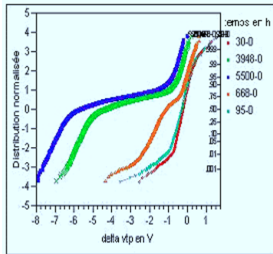
Figure 14 : Distribution de la variation de V_{TP} en fonction du temps à T=250^\circ\text{C} .
