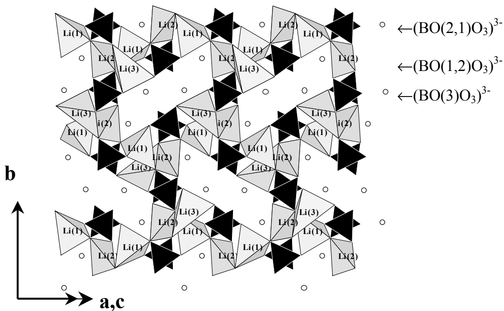
(Fig.1.1/7) Enchaînement des tétraèdres de coordination LiO 4 (Groupements (BO 3 ) 3- : triangles noirs, atomes de praséodyme : cercles vides)
