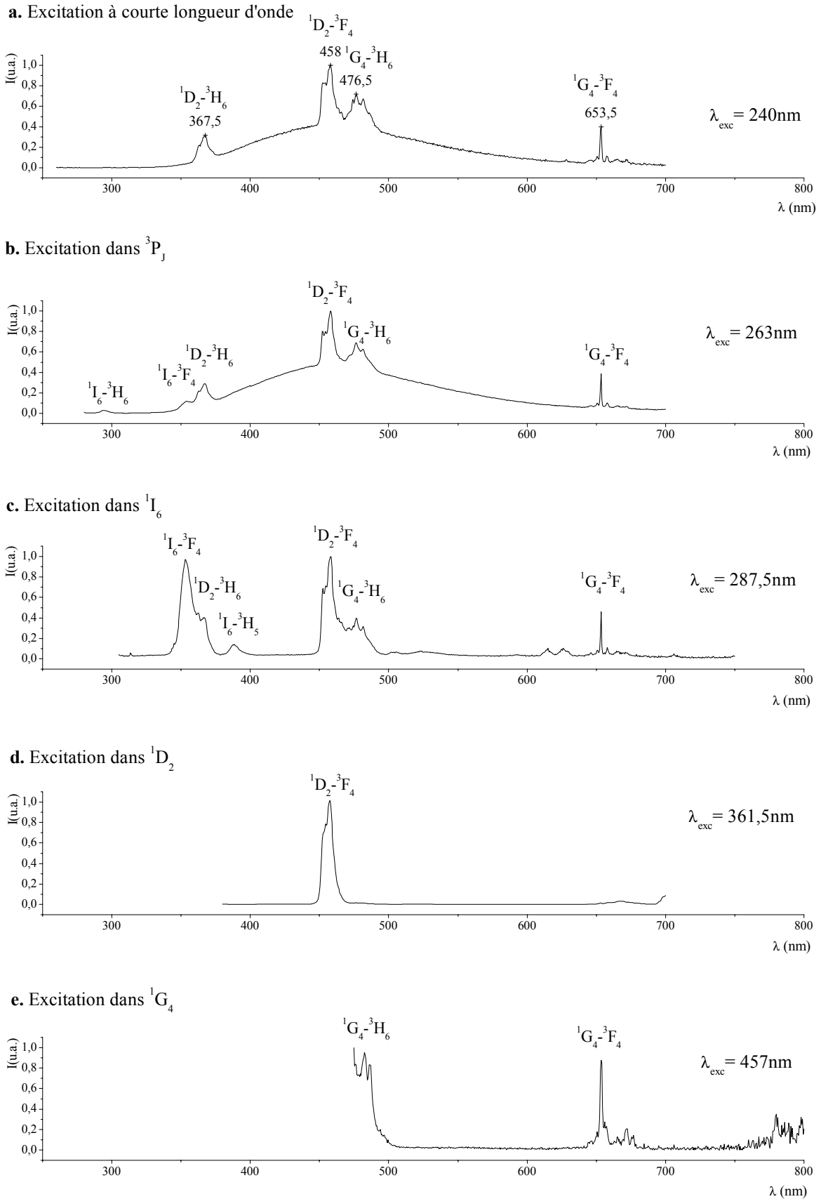
(Fig.2.4/6) Spectres d'émission de l'oxyborate \text{LiLa}_2\text{O}_2\text{BO}_3: \text{Tm}^{3+} 0,25\% à 300K.
