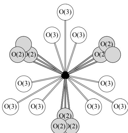
Projection dans le plan (001)
