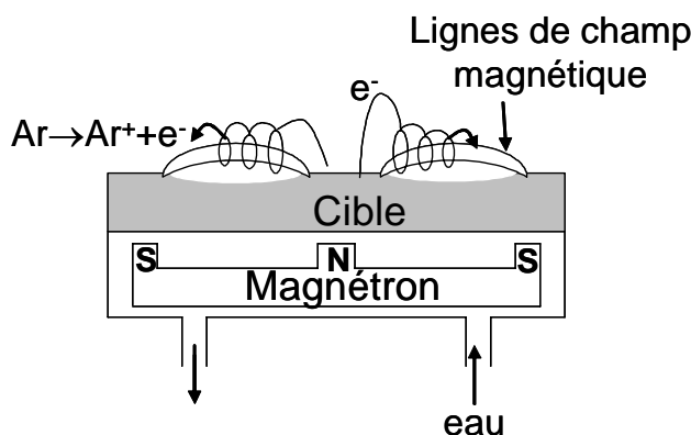
Figure II.5 : Schéma d'une cathode magnétron
