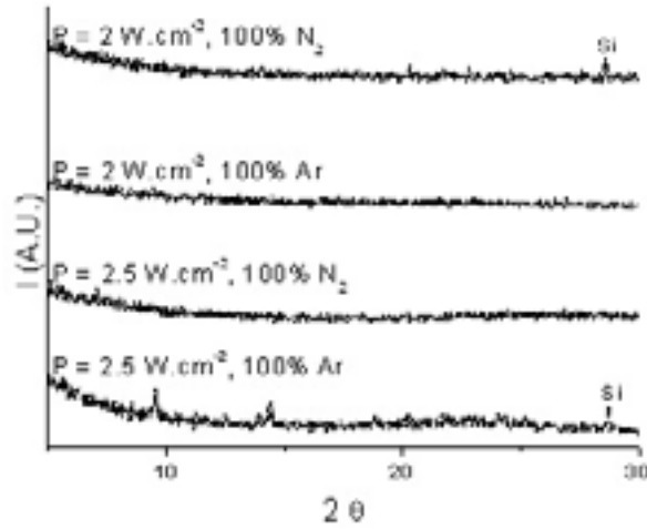
Figure V.12 : Diagramme de diffraction des rayons X des couches minces déposées avec une cible 0.14\text{B}_2\text{O}_3-0.21\text{Li}_2\text{O}-0.65\text{Li}_2\text{SO}_4
