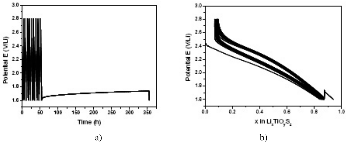
Figure III.35 : Cyclage d'une microbatterie tout solide avec la couche TiO_{0.6}S_{1.6} HEF 2 (O/S = 0.38) : évolution du potentiel en fonction a) du temps, b) du taux x de lithium inséré
