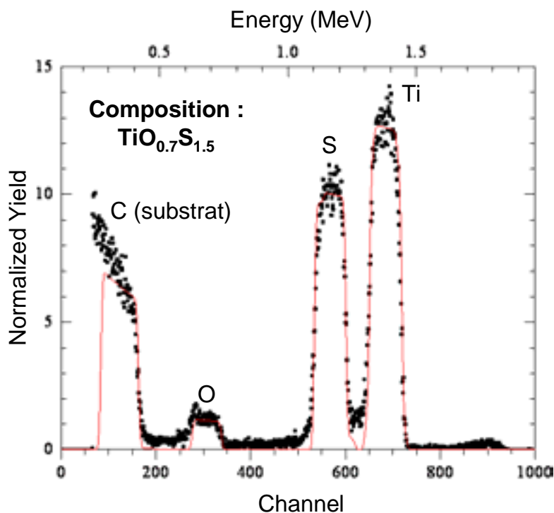
Figure II.11 : Spectre RBS expérimental d'une couche mince de composition \text{TiO}_{0.7}\text{S}_{1.5} (points) et sa simulation (trait plein)
