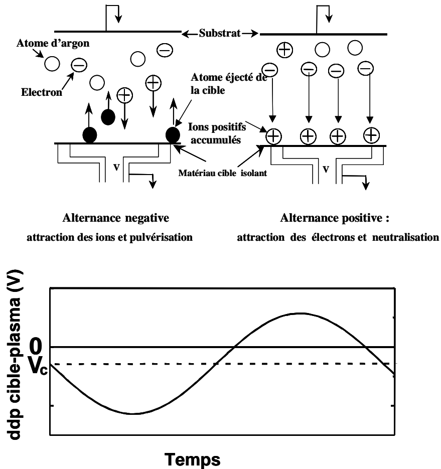
Figure II.4 : Principe de la pulvérisation cathodique radiofréquence
