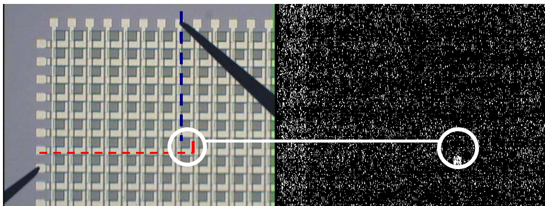
Figure IV-8 : Test électrique et validation de l'adressage de puissance par visualisation de l'élément sélectionné.
