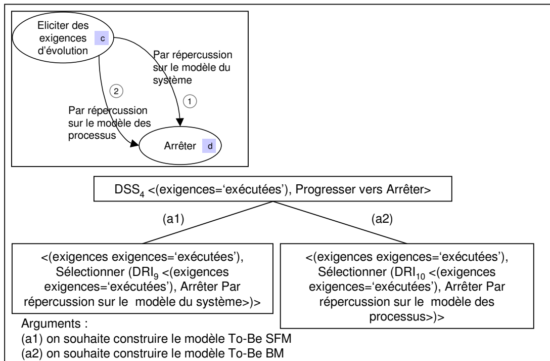
Figure 121 : Directive de sélection de stratégie permettant de progresser vers Arrêter
