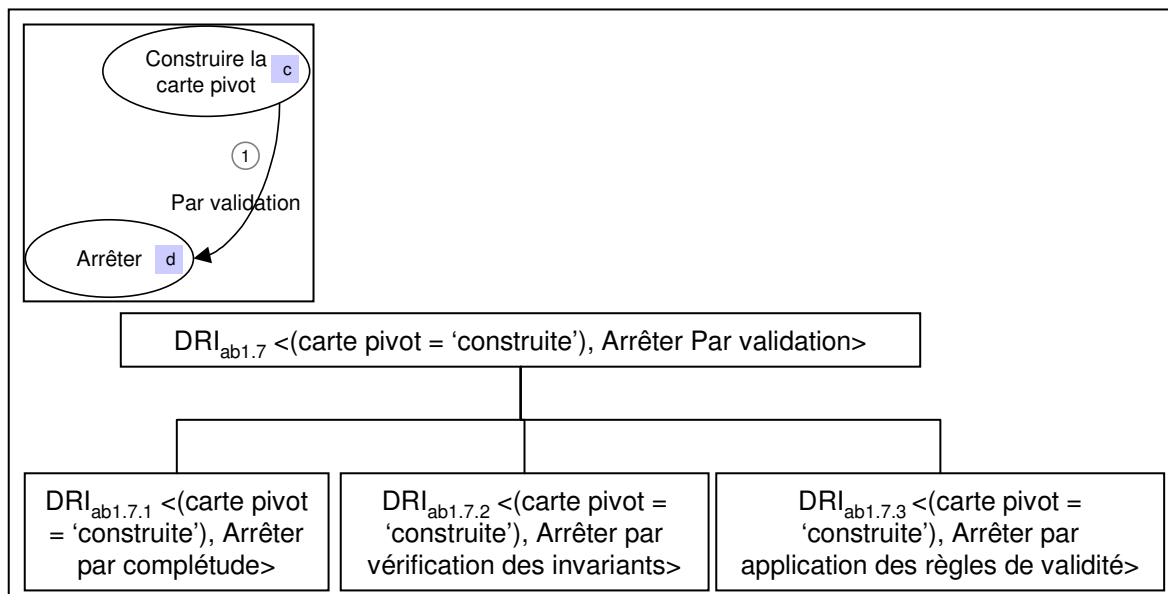
Figure 107 : Directive plan permettant d'Arrêter Par validation le processus de construction du modèle pivot
