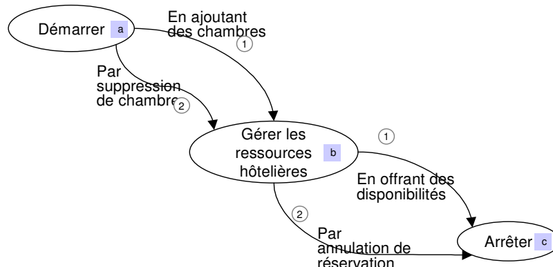
Figure 125 : Carte Cs ab2 décrivant l'offre d'un produit par modification de ressources
