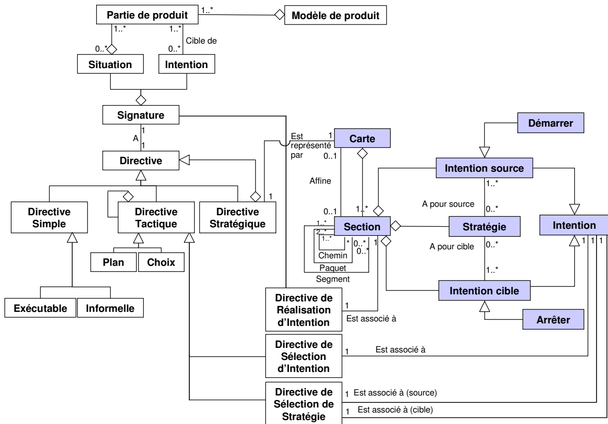
Figure 70 : Méta-modèle de Carte vu comme méta-modèle de processus
