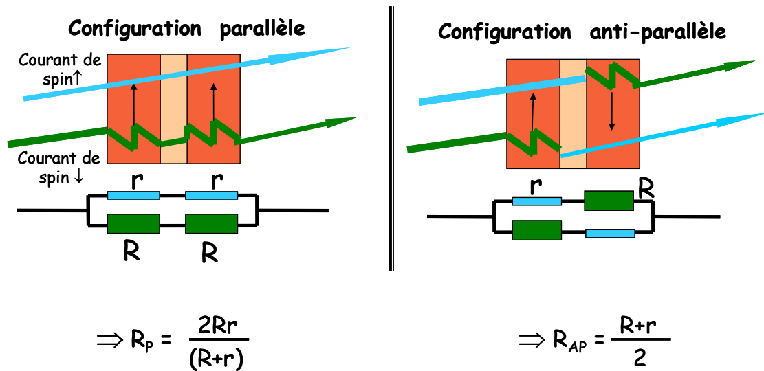
Figure IV-5 : Différence de résistivité entre un état parallèle et un état anti-parallèle.
