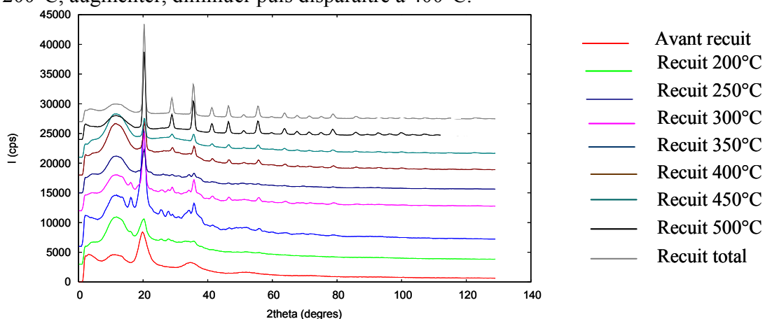
Figure III-6 : Diffractogrammes de NMI à différentes températures de recuit.
