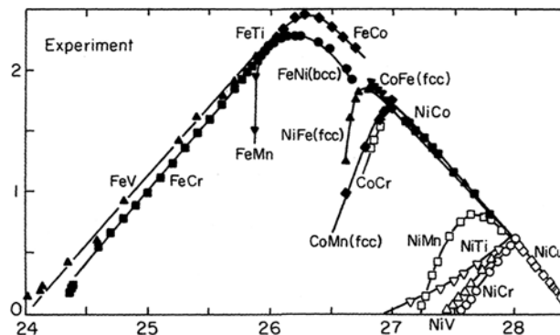
Figure I-3 : moment magnétique de l'alliage ( \mu_B/at ) en fonction du nombre d'électrons par atome. [6]
