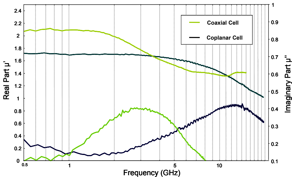
Figure IV-23 : Evolution de la perméabilité de NMI en fonction de la fréquence par la méthode coplanaire (noir) et coaxiale (vert).
