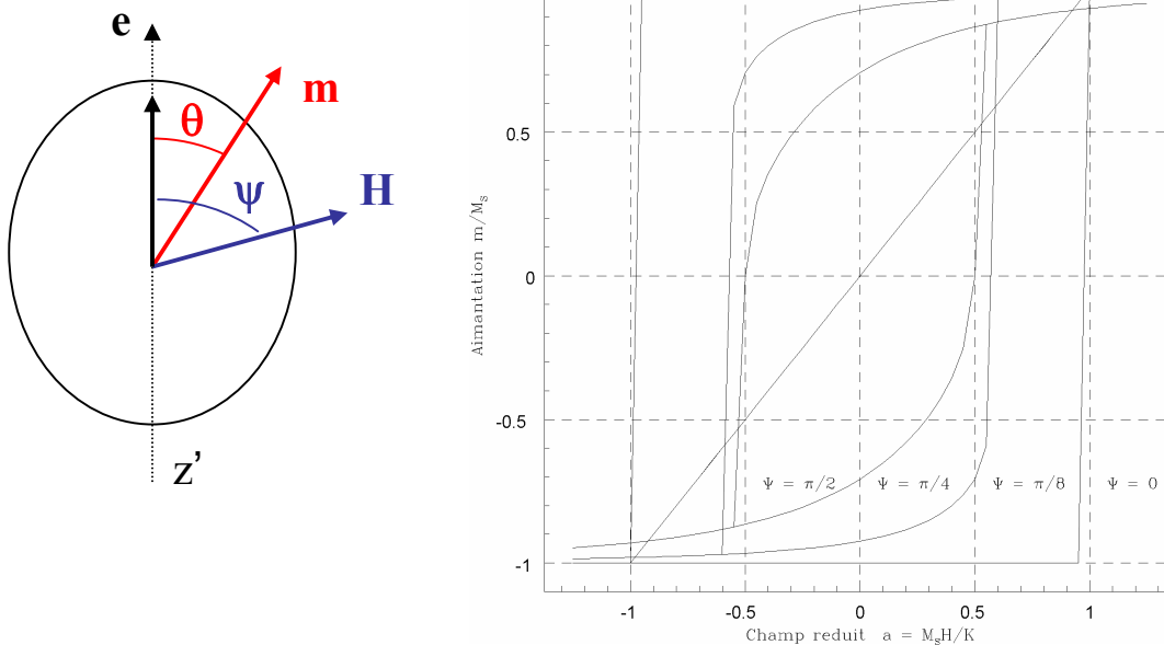
Figure 1-7 : Courbe d'hystérésis dans le modèle de Stoner-Wohlfarth pour différentes orientations du champ magnétique par rapport à l'axe d'anisotropie
