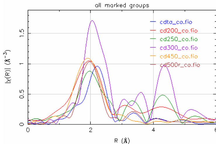
Figure III-11 : Spectres EXAFS au seuil du cobalt de NMI aux différentes températures de recuit.
