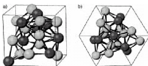
Figure I-9 : Motif unitaire du cobalt- \epsilon : a) cube unitaire composé de 8 atomes de cobalt dans une configuration I (noir) et de 12 atomes de cobalt dans une configuration II (gris) ; b) projection 111 du même cube montrant la symétrie le long de la grande diagonale. [29]
