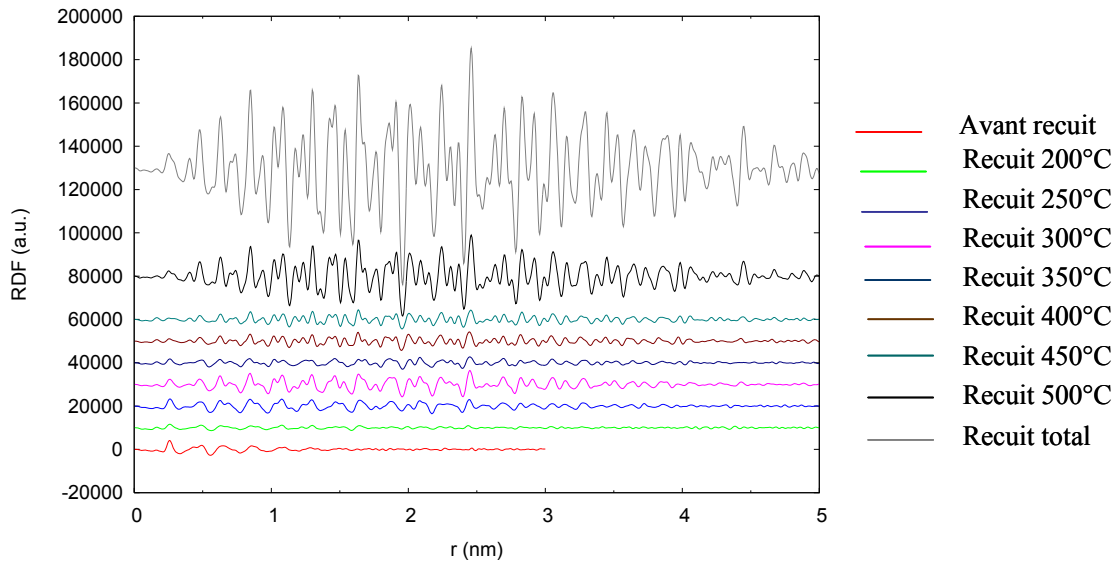
Figure III-7: RDF NMI à différentes température de recuit. CD66 : NMI avant recuit, CD66R : NMI après recuit total.
