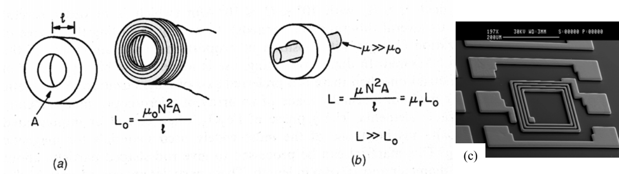
Figure I- 1 : a ) Inducteur classique; b) inducteur en présence d'un matériau magnétique ;c) photo d'une série d'inducteurs utilisés en microélectronique.
