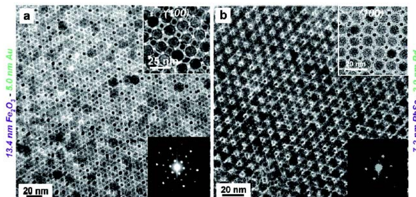
Figure I-15 : Exemple de métamatériaux : Fe_3O_4Au et PbSePd . [113]
