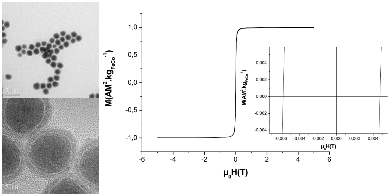
Figure II-15 : a) NMI après 2 semaines d'exposition à l'air : gris foncé : cœur métallique, gris clair : oxyde ; b) Hystérésis à 2K après refroidissement sous 5T : décalage du cycle d'hystérésis dû à l'oxydation.
