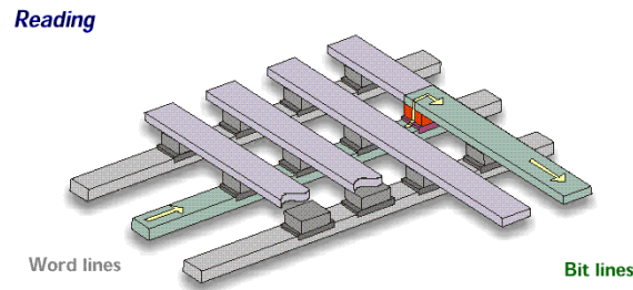
Figure IV-2 : Schéma d'une MRAM.
