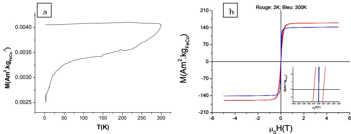
Figure II-3 : Propriétés magnétiques de NMI : a) ZFC/FC ; b) hystérésis à 2K (rouge) et à 300K (bleu).
