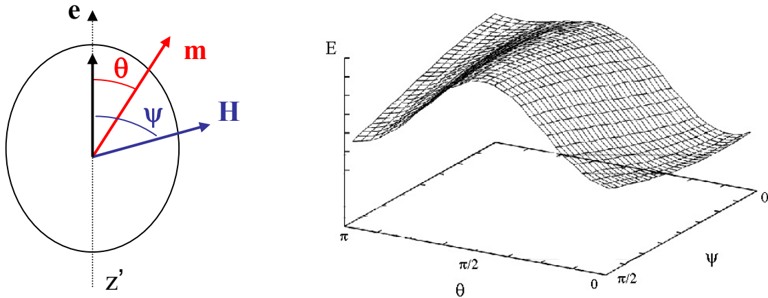
Figure A1-6 : Particule dans le modèle de Stoner-Wolfarth et surface d'énergie
