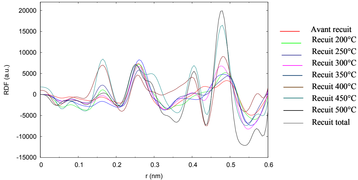
Figure III-9: Agrandissement normalisé des RDF NMI à différentes température de recuit.
