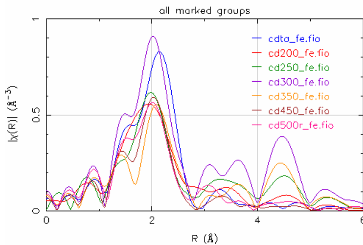
Figure III-10 : Spectres EXAFS au seuil du fer de NMI aux différentes températures de recuit.
