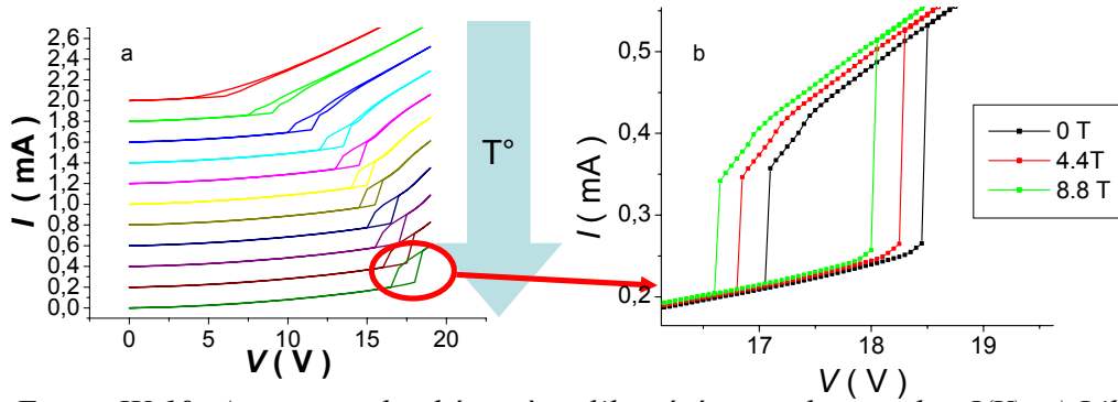
Figure IV-19: Apparition du phénomène d'hystérésis sur les courbes I(V) . a) L'hystérésis se décale vers la droite lorsque T diminue ; b) Décalage de l'hystérésis vers la gauche lorsque le champ magnétique augmente.
