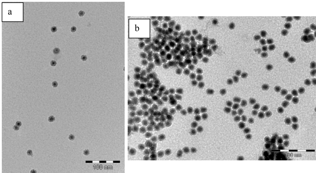
Figure III-18 : Clichés TEM des particules stabilisé par H_3PO_4 et enrobées d'une couche de SiO_2 : a) après 3 jours, la couche de silice se forme ; b) après 10 jours les particules sont enrobées de SiO_2 .
