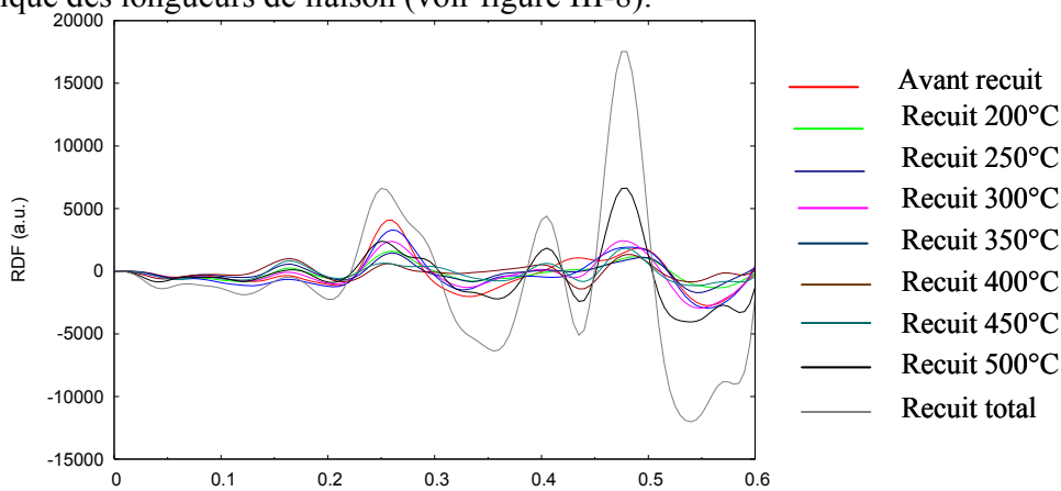
Figure III-8: Agrandissement sur les petites distances des RDF NMI à différentes température de recuit. CD66 : NMI avant recuit, CD66R : NMI après recuit total.
