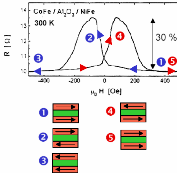
Figure IV-6 : Courbe expérimentale de la TMR dans un matériau CoFe/Al 2 O 3 /NiFe.
