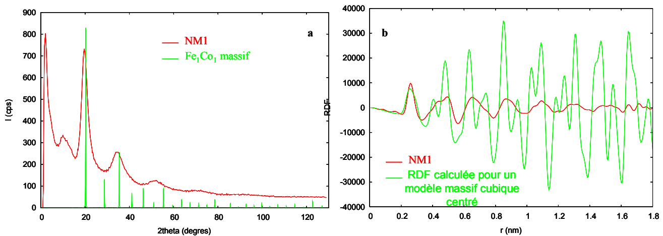
Figure II-9 : Etude WAXS de NMI : a) diffractogramme de NMI et comparaison avec les pics attendus pour un alliage de Fe 1 Co 1 ; b) RDF de NMI et comparaison avec la RDF calculée pour un modèle cubique centré.
