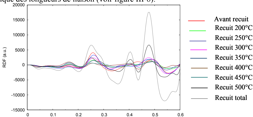
Figure III-8: Agrandissement sur les petites distances des RDF NMI à différentes température de recuit. CD66 : NMI avant recuit, CD66R : NMI après recuit total.
