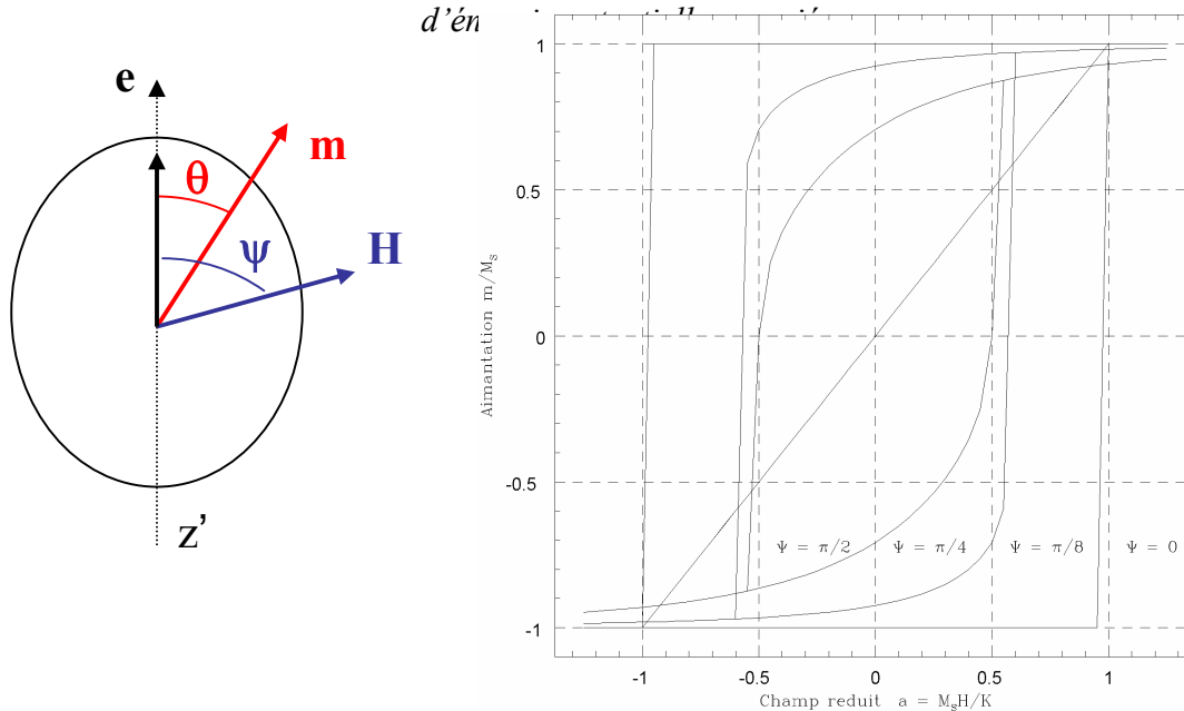
Figure 1-7 : Courbe d'hystérésis dans le modèle de Stoner-Wolfarth pour différentes orientations du champ magnétique par rapport à l'axe d'anisotropie
