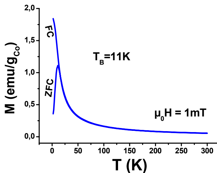
Figure A1-5 : Courbes ZFC/FC de nanoparticules avec distribution de taille.
