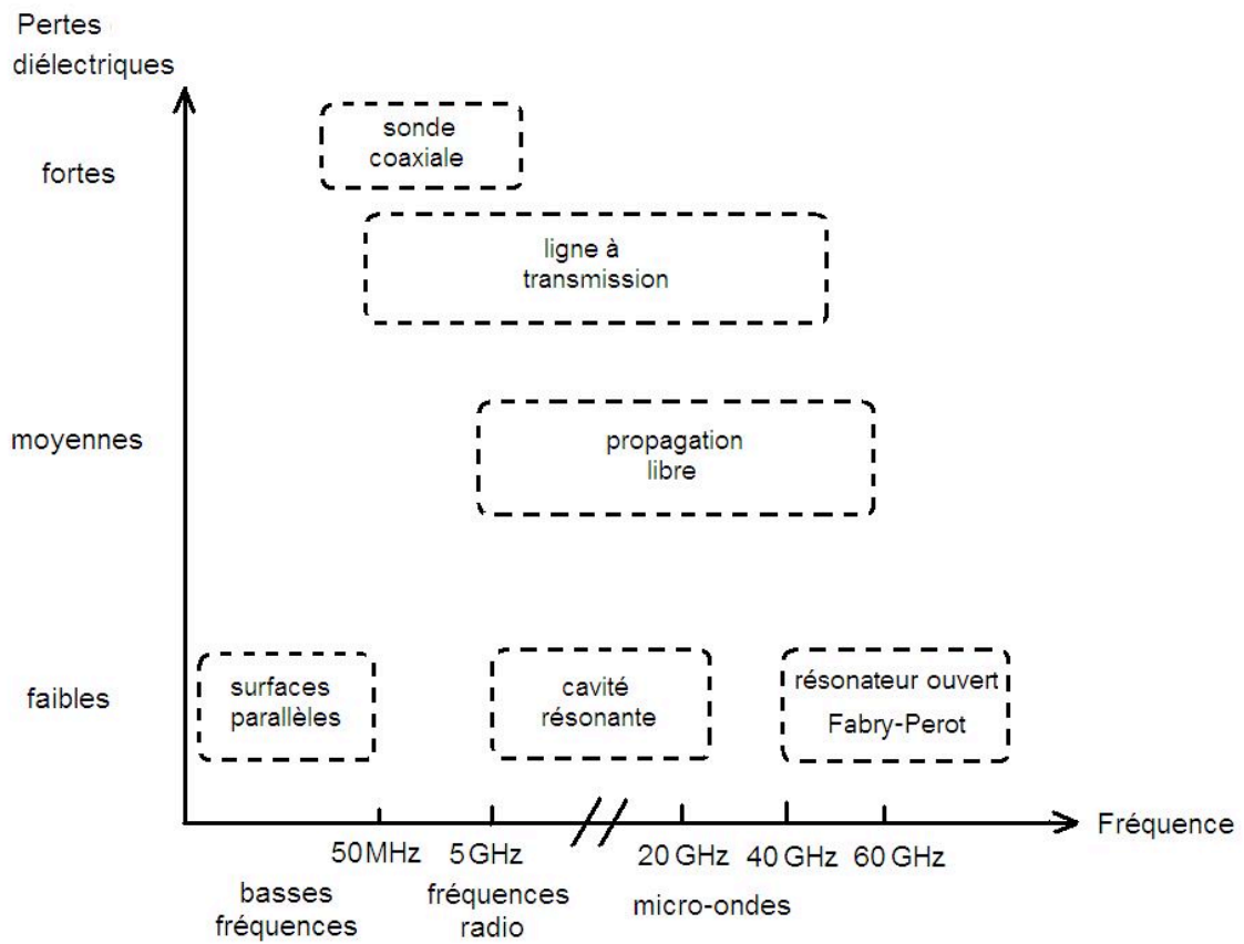
Figure 5-28 : Bandes de fréquences et gammes de pertes diélectriques associées aux différentes méthodes de mesure de permittivité diélectrique.
