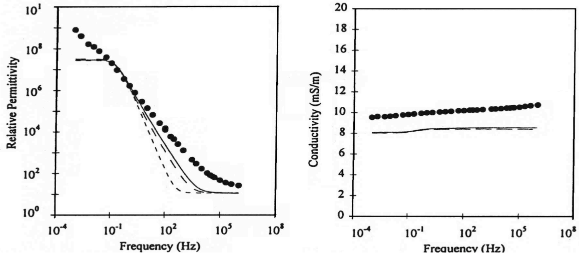
Figure 4-40 : Comparaison des réponses modélisées avec la distribution de volume des grains extrapolée et des réponses mesurées pour le grès Bêrea (points). Comparaison de différentes formules :
