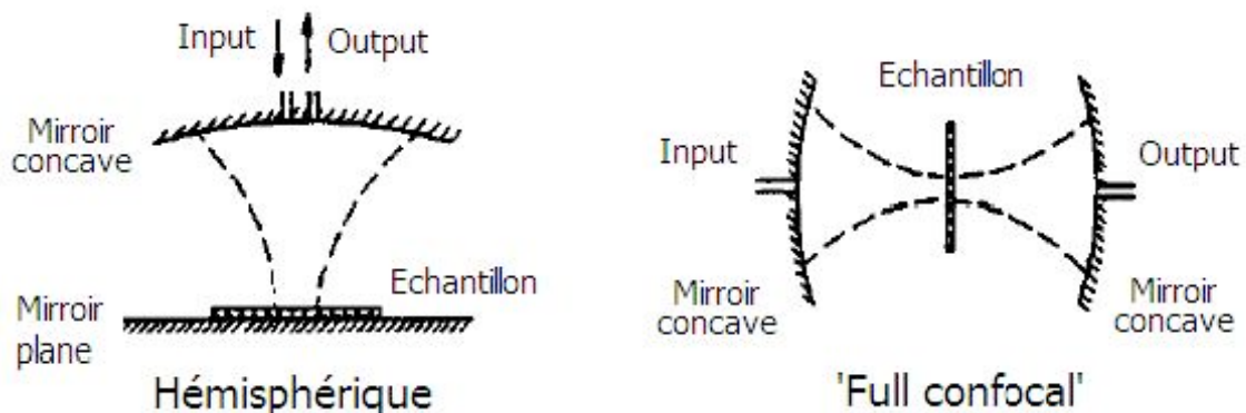
Figure 5-15 : Schéma d'une cavité résonante de type résonateur ouvert de Fabry-Perot. À gauche : dispositif hémisphérique ; à droite : dispositif « full confocal ». La constante diélectrique et la tangente de pertes sont déduites des variations de la fréquence de résonance du système et du facteur de qualité.
