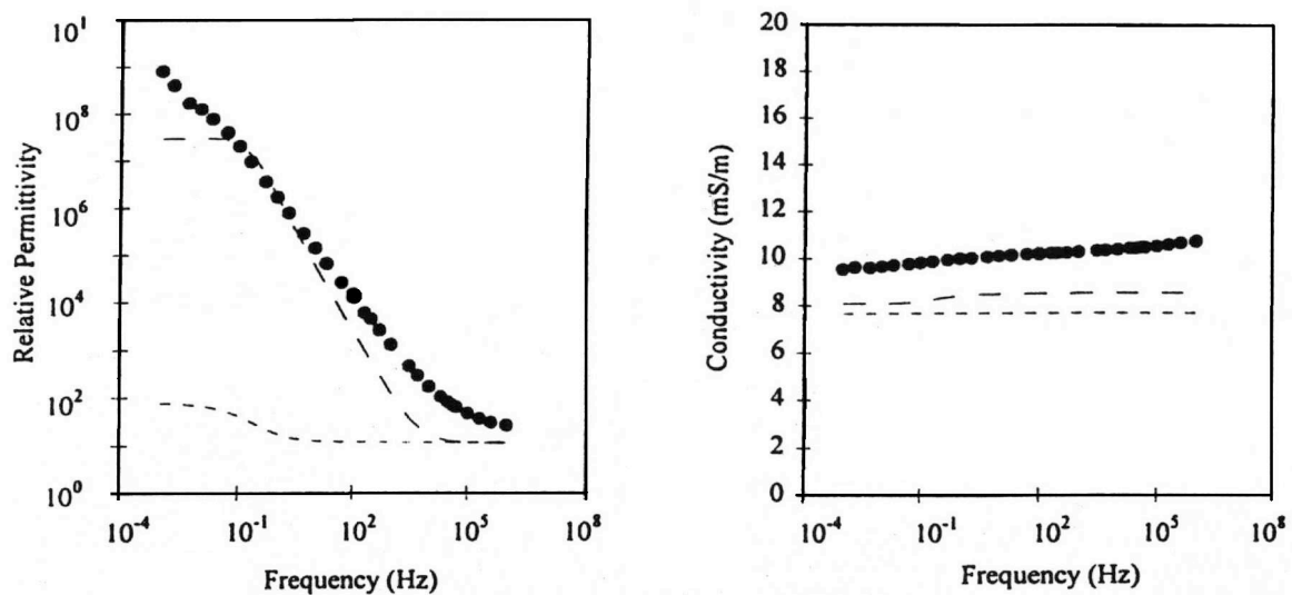
Figure 4-41 : Comparaison des réponses modélisées avec la distribution de volume des grains extrapolée avec la formule de mélange en parallèle, et des réponses mesurées pour le grès Bêrea (points) : Contribution de la polarisation de la couche fixe — — —
