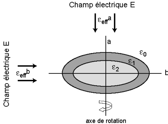
Figure 4-27 : Géométrie correspondant à un système avec des ellipsoïdes concentriques (de propriétés \epsilon_1 et \epsilon_2 ), plongés dans une troisième phase ( \epsilon_0 ).
