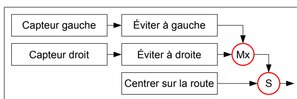
Figure II.10 : Modèle de navigation basé sur l'AFAG.
