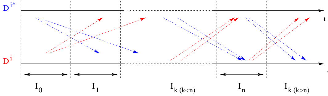
FIG. 2.5 – Décomposition de l'intervalle d'étude à l'aide du principe de Huygens, et répartition des interactions entre les domaines
