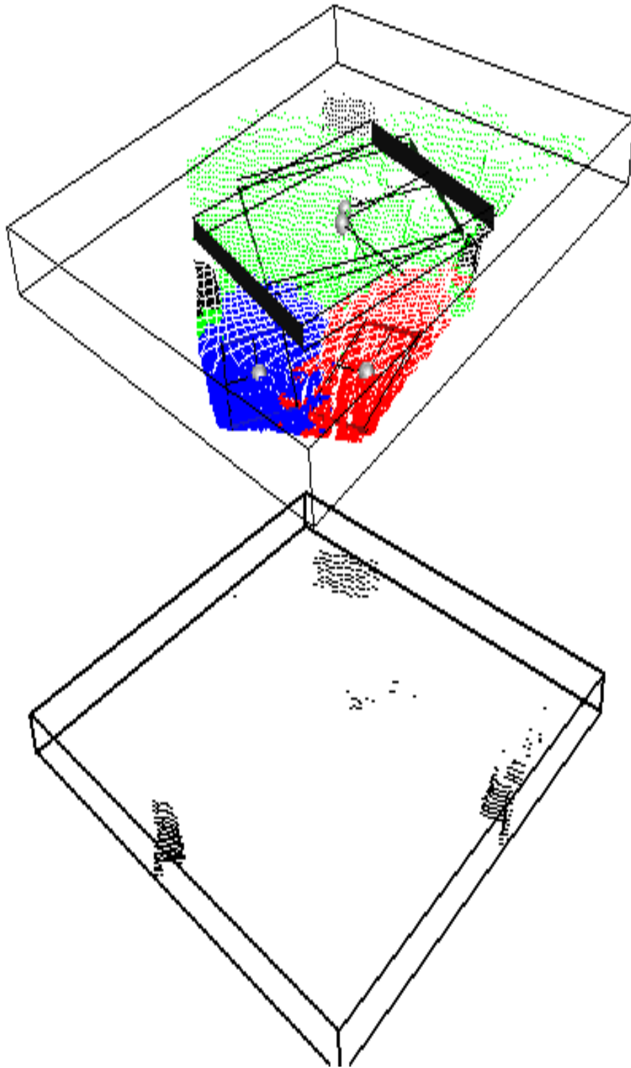
FIG. 6.5 – Au-dessus 4-partition dans laquelle trois rochers de structure ellipsoïdale émergent dans un groupement de couleur noire d'une large zone planaire de couleur verte et sont rassemblés dans un seul groupement ; en-dessous l'objet posant problème isolé
