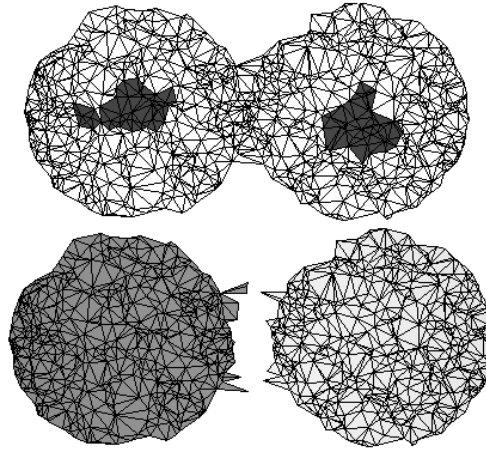
FIG. 5.7 – De haut en bas : 0.8-ouverture d'ordre 7 ; Dilatation géodésique des deux germes
