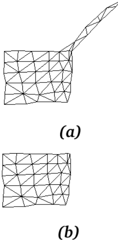
FIG. 5.3 – Filtrage de la forme (a) par ouverture d'ordre 1 (b)
