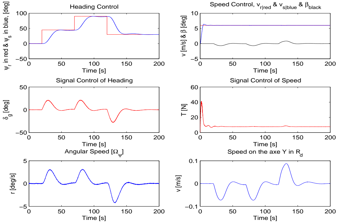
FIG. 3.18 – Control de dirección en el plano horizontal, regulador NL-PO
