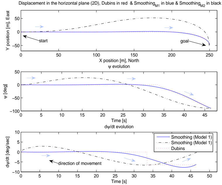
FIG. 4.2 – Trayectoria de vuelo para el dirigible, \zeta_i = [0, 0, 0] y \zeta_f = [250, -250, -90]
