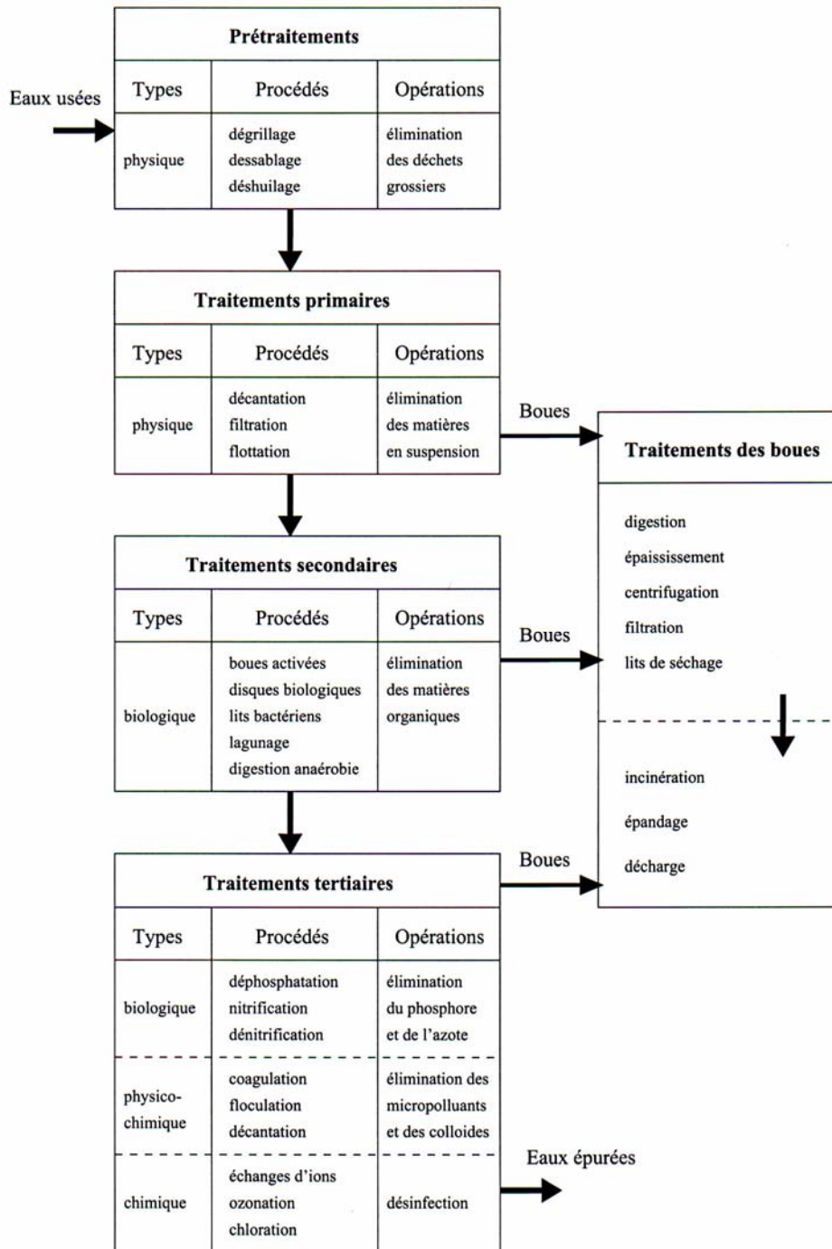
Figure 1.1. Filière d'épuration des eaux résiduelles (d'après [HAD99]).
