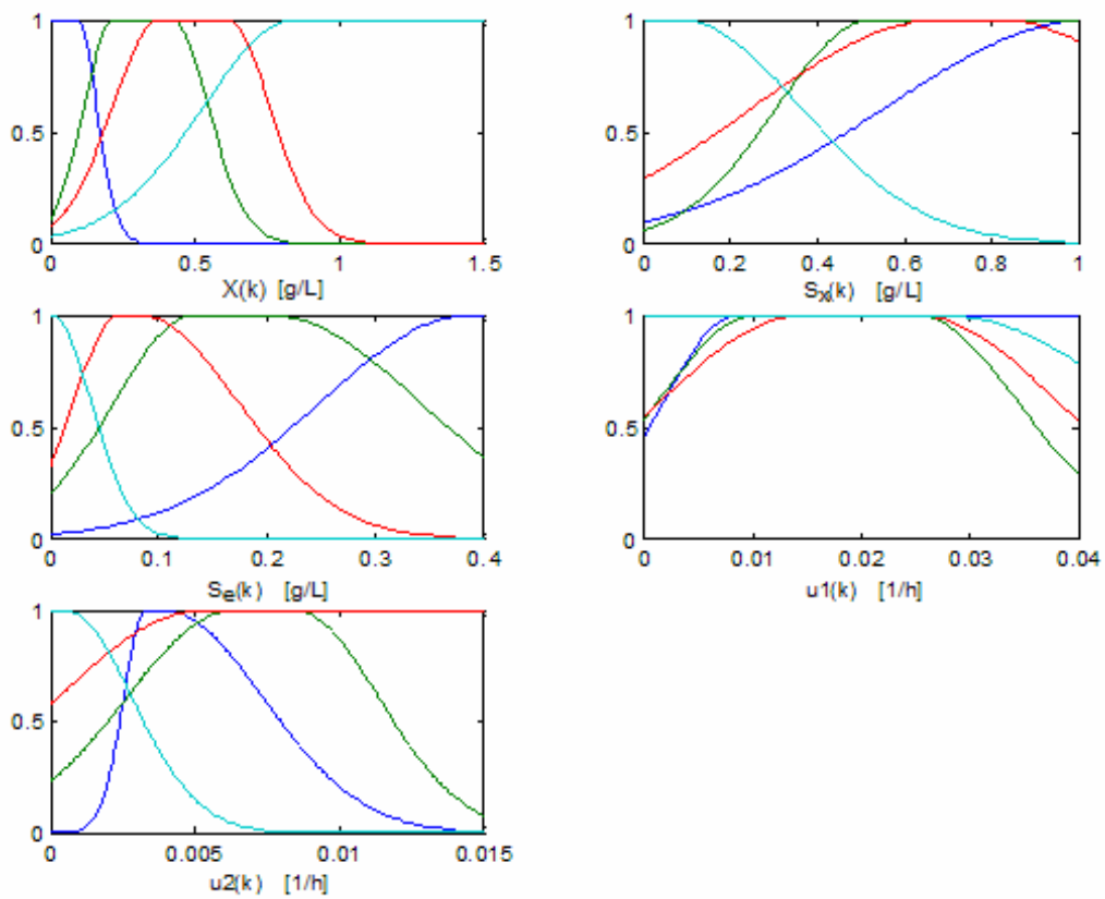
Figure 5.10. Partition S_x(k) avec GK données d'opération en mode continu
