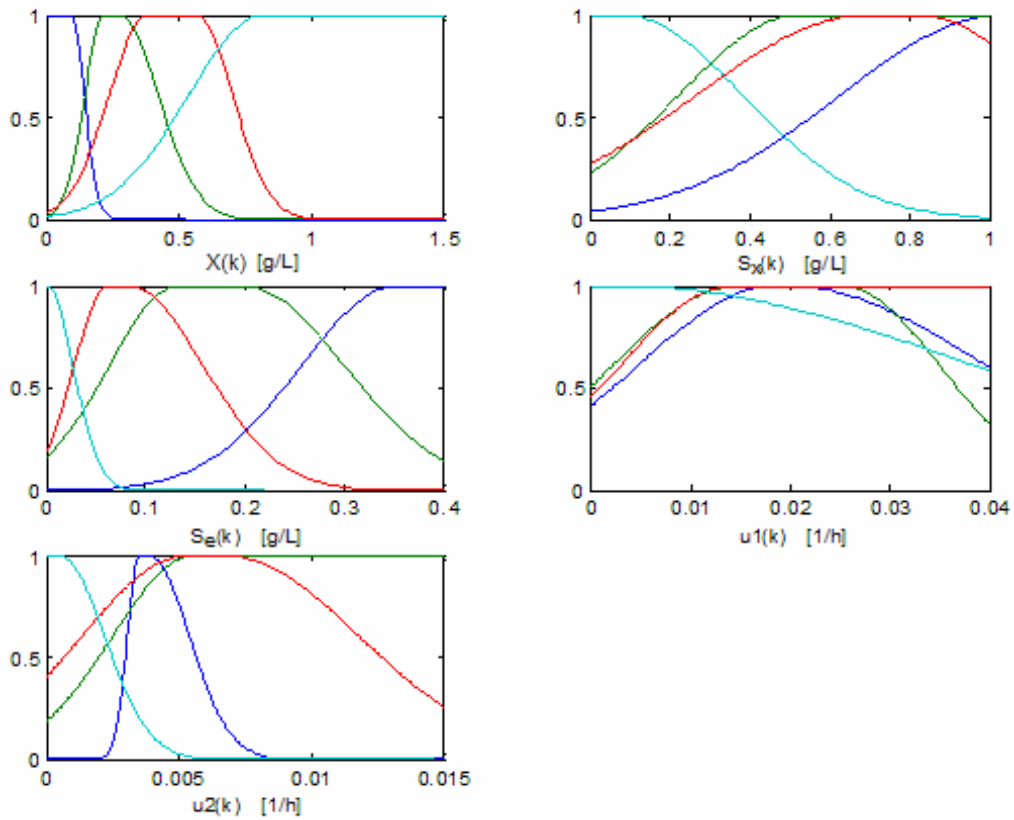
Figure 5.11. Partition S_e(k) avec GK données d'opération en mode continu
