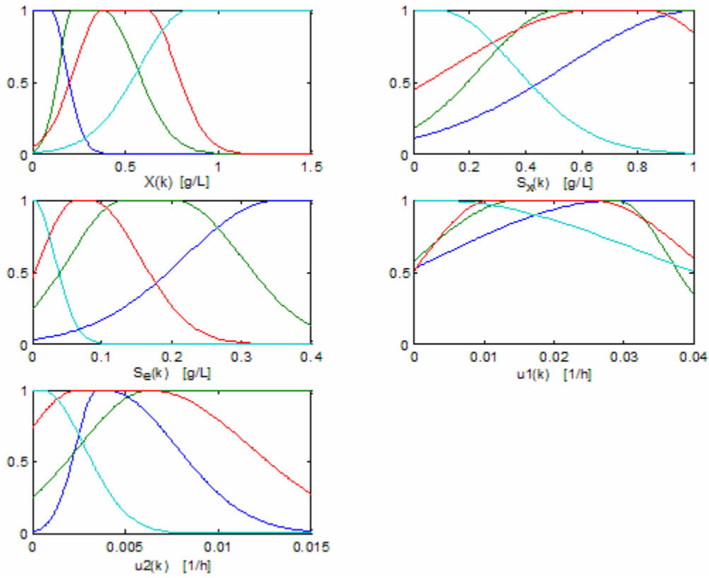
Figure 5.9. Partition X(k) avec GK données d'opération en mode continu
