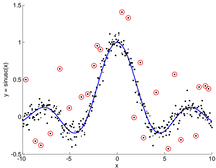
Figure 3.11. Fonction y(x) = \text{sinusc}(x) avec bruit et points aberrants (cercles)
