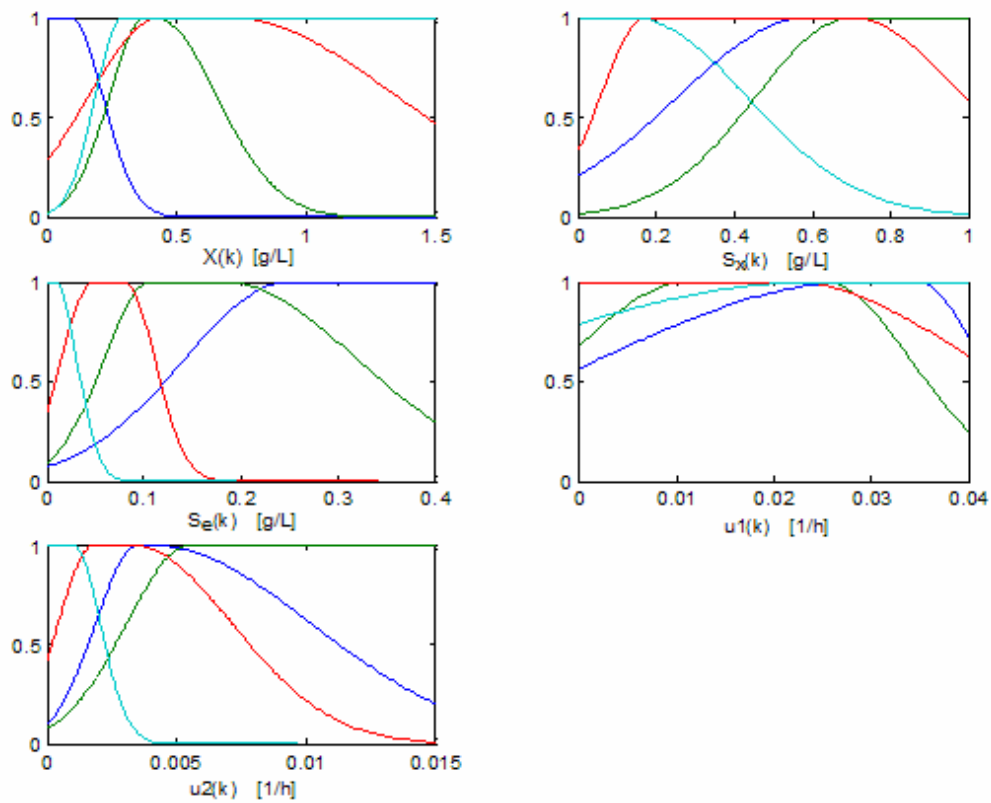
Figure 5.12. Partition X(k) avec RoFER données d'opération en mode continu
