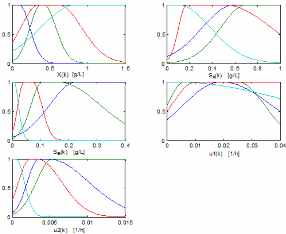
Figure 5.14. Partition S_e(k) avec RoFER données d'opération en mode continu
