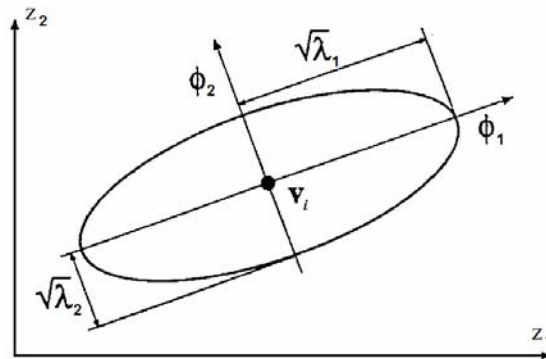
Figure 3.4. Interprétation géométrique de la matrice de covariance floue (d'après [BAB98a]) L'équation (\mathbf{z}-\mathbf{v})^T \mathbf{F}^{-1} (\mathbf{z}-\mathbf{v}) = 1 définit un hyperellipsoïde dans \mathfrak{R}^n .
