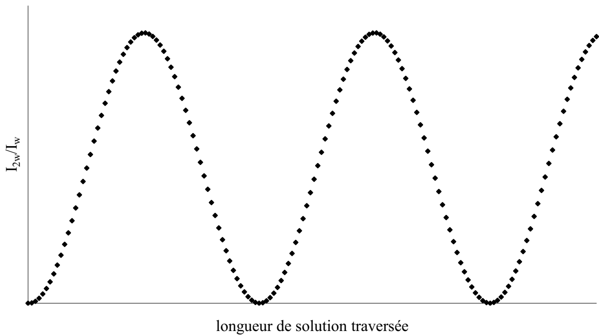
Fig. 4 : Franges de Maker générées par la variation de la longueur de solution traversée
