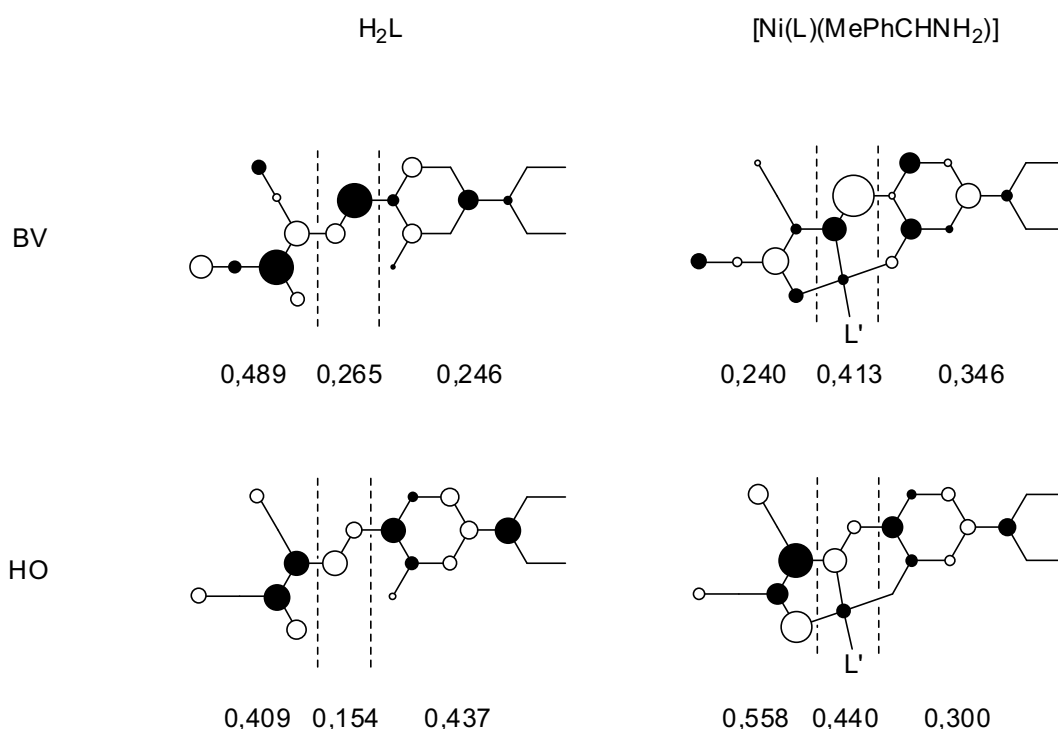
Fig. 6 : Densité électronique des orbitales frontières de H 2 L et [Ni(L)MePhCHNH 2 ]. Les nombres indiquent la part de la densité sur chaque fragment.
