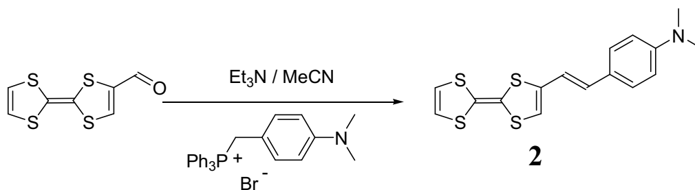
Fig. 8 : Voie de synthèse du composé 2
