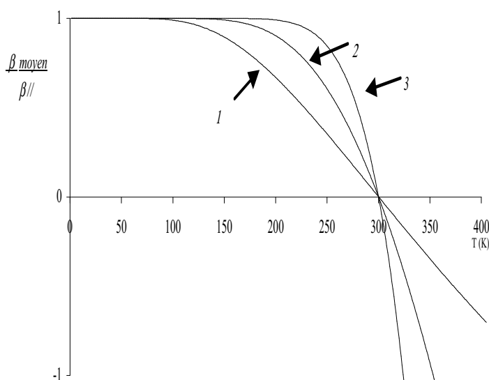
Fig. 10 : Dépendance en température du \beta moyen relatif (exprimé comme \beta_{moyen} / \beta_{\parallel} ), pour des barrières d'énergie égales à 1,4 (1), 2,8 (2), et 5,6 (3) kcal.mol -1
