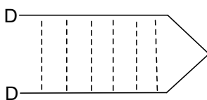
Fig. 14 : Représentation schématique de 2 tétrathiafulvalènes reliés par un lien chimique
