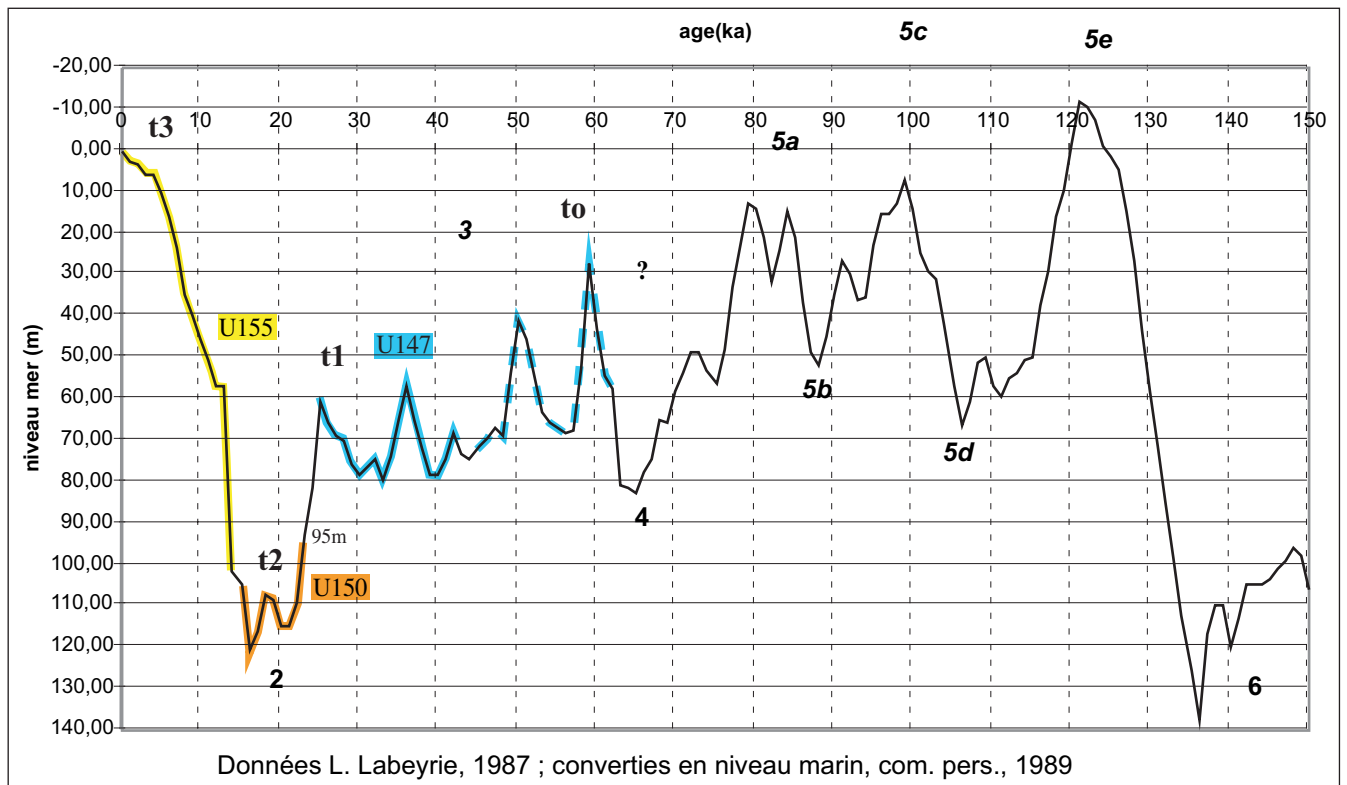
Figure V-2 Corrélation des unités U147, U150 et U155 avec la courbe de variations du niveau marin. En trait plein : portion d'unité directement prélevée ; en tirets : extrapolation. t0 et t3 correspondent au temps indiqué sur les figures V-4 et V-5 ; t0 : début du stade 3 ; t1 : fin du stade 3 et début du stade 2 ; t2 : fin du stade 2 ; t3 : stade 1 (actuel).
