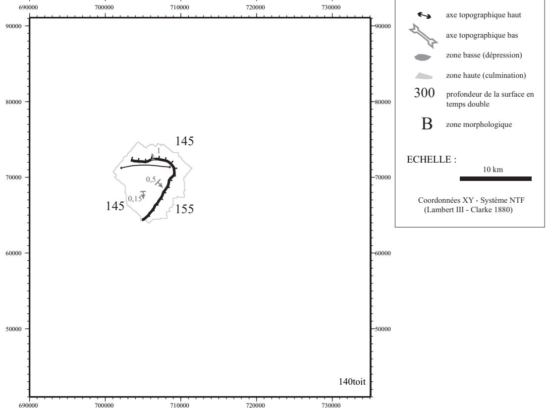
Figure III-37B Interprétation de la carte isohypse temps double : principaux traits morphologiques de la surface U140 Toit (Voir carte original en Annexe C).
