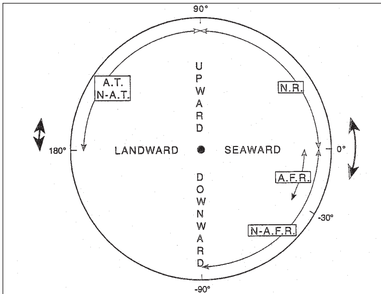
Figure I-16 Cercle de trajectoire de la ligne de rivage. Les flèches à l'extérieur du cercle indiquent les trajectoires les plus fréquentes. AFR : Régression forcée en accréation ; NAFR : Régression forcée non-en-accréation ; NR : Régression normale ; AT : Transgression en accréation ; NAT : Transgression non-en-accréation (Helland-Hansen, 1996).
