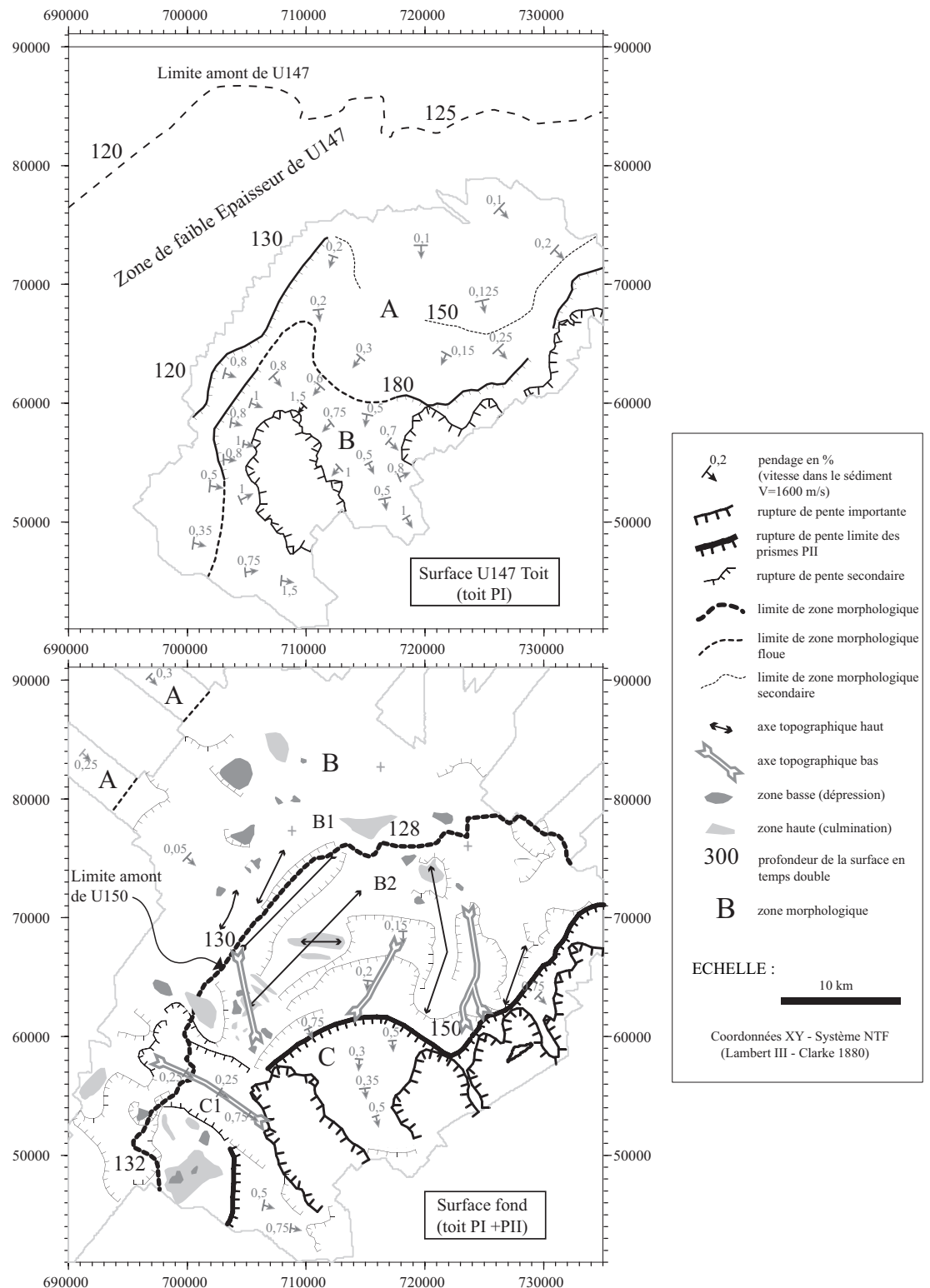
Figure III-40A Interprétation de la carte isohypse temps double : principaux traits morphologiques de la surface U147 Toit (voir carte en Annexe C).
