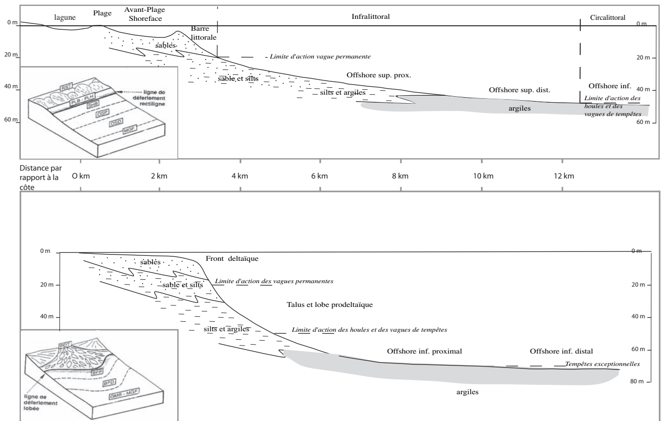
Figure II-28 Comparaison de 2 types de profils bathymétriques réels du Golfe du Lion : compilation d'après des données bathymétriques et des descriptions sédimentologiques (Aloisi, 1986 ; Bruzzi, 1998 ; les diagrammes en 3D sont empruntés à Lafont, 1994 ; RST : replat sableux à débordement de tempêtes ; PLB-PLH : Plage ; SHB : avant-plage ; OSP et OSD : offshore supérieur proximal et distal ; MGF : offshore inférieur ; BFP-BFD : front de delta proximal et distal.
