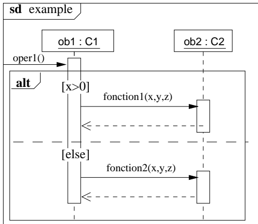
FIG. 5.3: Message dans le diagramme de séquence
