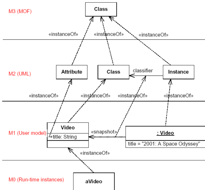
FIG. 1.2: Exemple de la hiérarchie de méta-modélisation en 4 couches
