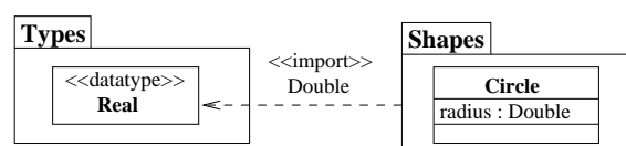
FIG. 5.22: Importation d'élément avec alias
