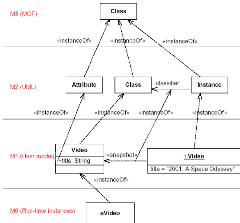
FIG. 1.2: Exemple de la hiérarchie de méta-modélisation en 4 couches
