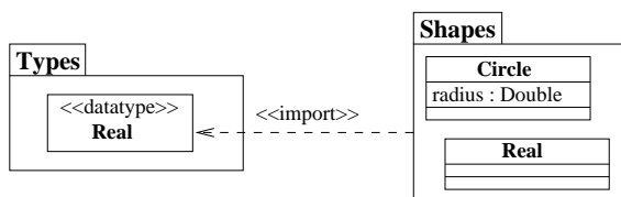
FIG. 5.21: Importation d'élément sans alias
