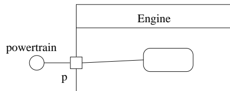
FIG. 5.31: Représentation d'un port comportemental
