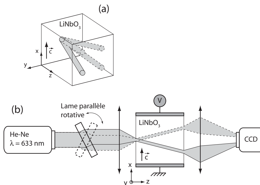
FIG. 4.6 : (a) Principe du connecteur 3-D 1 × 4 et (b) schéma du dispositif expérimental correspondant.
