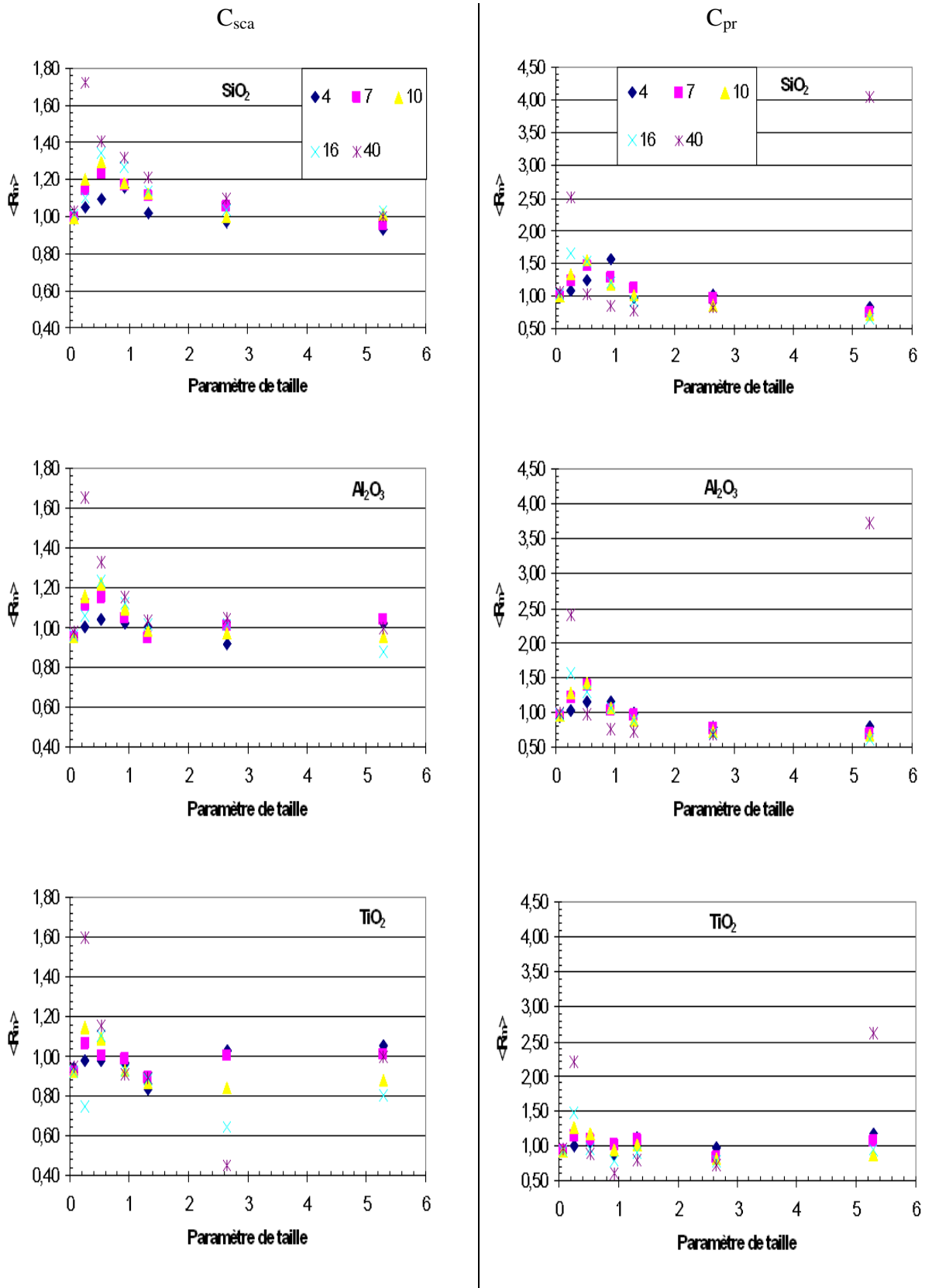
Figure B- VI-11 : C_{\text{sca}} et C_{\text{pr}} d'agrégats (de 4, 7, 10, 16 ou 40 particules primaires) construits suivant le mécanisme BCCA pour des matériaux ( \text{SiO}_2 , \text{Al}_2\text{O}_3 et \text{TiO}_2 ) ayant un indice de réfraction réel.
