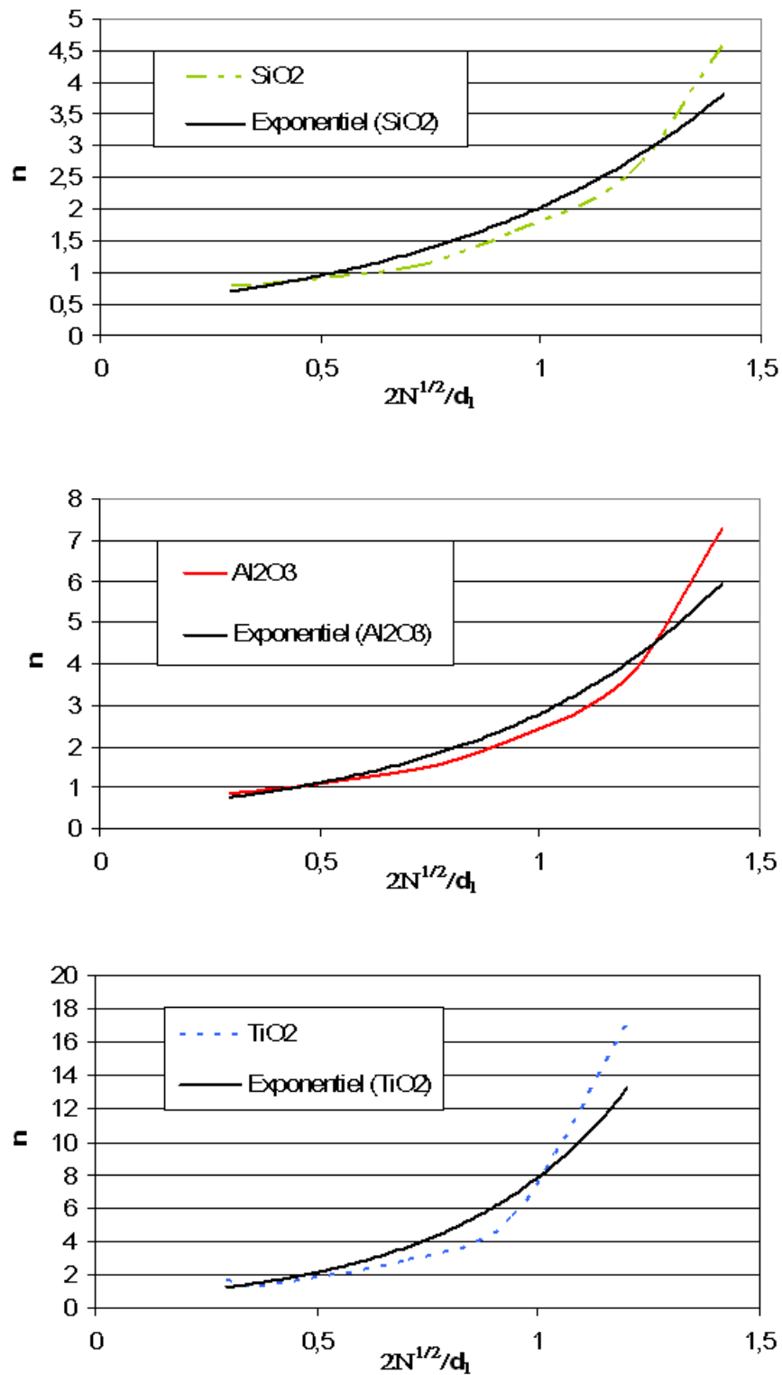
Figure B- VI-6: Evolution de n en fonction de d_1 et N pour les trois matériaux ( \text{SiO}_2 , \text{Al}_2\text{O}_3 , \text{TiO}_2 )
