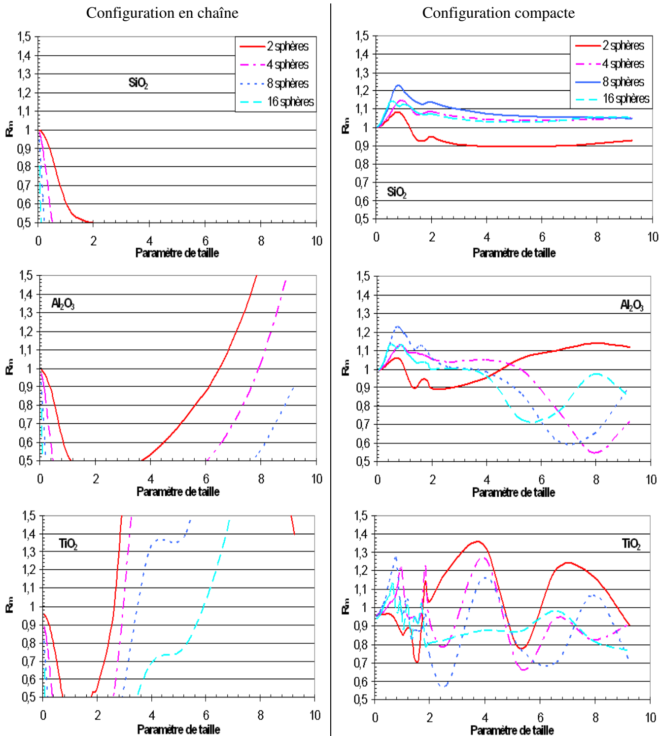
Annexe Figure 12: Méthode Fractal : Avec R_m \in [0.5, 1.5] en fonction du paramètre de taille, pour les 3 matériaux (SiO 2 , Al 2 O 3 , TiO 2 ) et suivant 2 configurations : en chaîne (1 ière colonne) et compacte (2 ième colonne).
