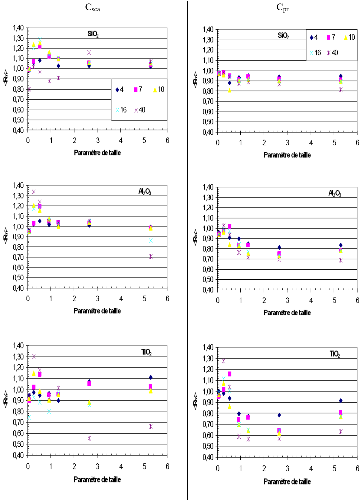
Figure B- VI-14 : C_{sca} et C_{pr} d'agrégats (de 4, 7, 10, 16 ou 40 particules primaires) construits suivant le mécanisme BCCA pour des matériaux ( SiO_2 , Al_2O_3 et TiO_2 ) ayant un indice de réfraction complexe.
