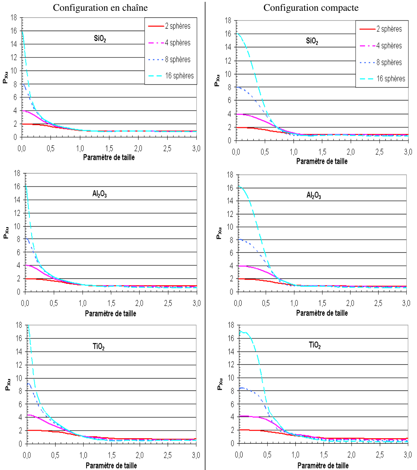
Annexe Figure 2: idem que Figure B- III-12 (page - 132 -) mais pour un paramètre de taille maximal de 3
