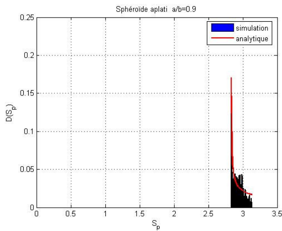
Figure B- I-7: Distribution des surfaces projetées S_p pour un sphéroïde de type aplati
