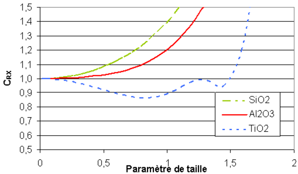
Annexe Figure 9: Domaine de validité de l'approximation de Rayleigh pour une sphère pour les 3 matériaux ( SiO_2 , Al_2O_3 , TiO_2 ).
