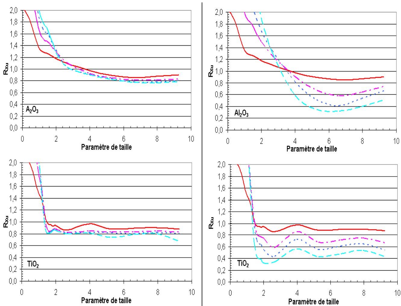
Figure B- III-4: idem que la Figure B- III-2 mais avec R_{xu} entre 0 et 2
