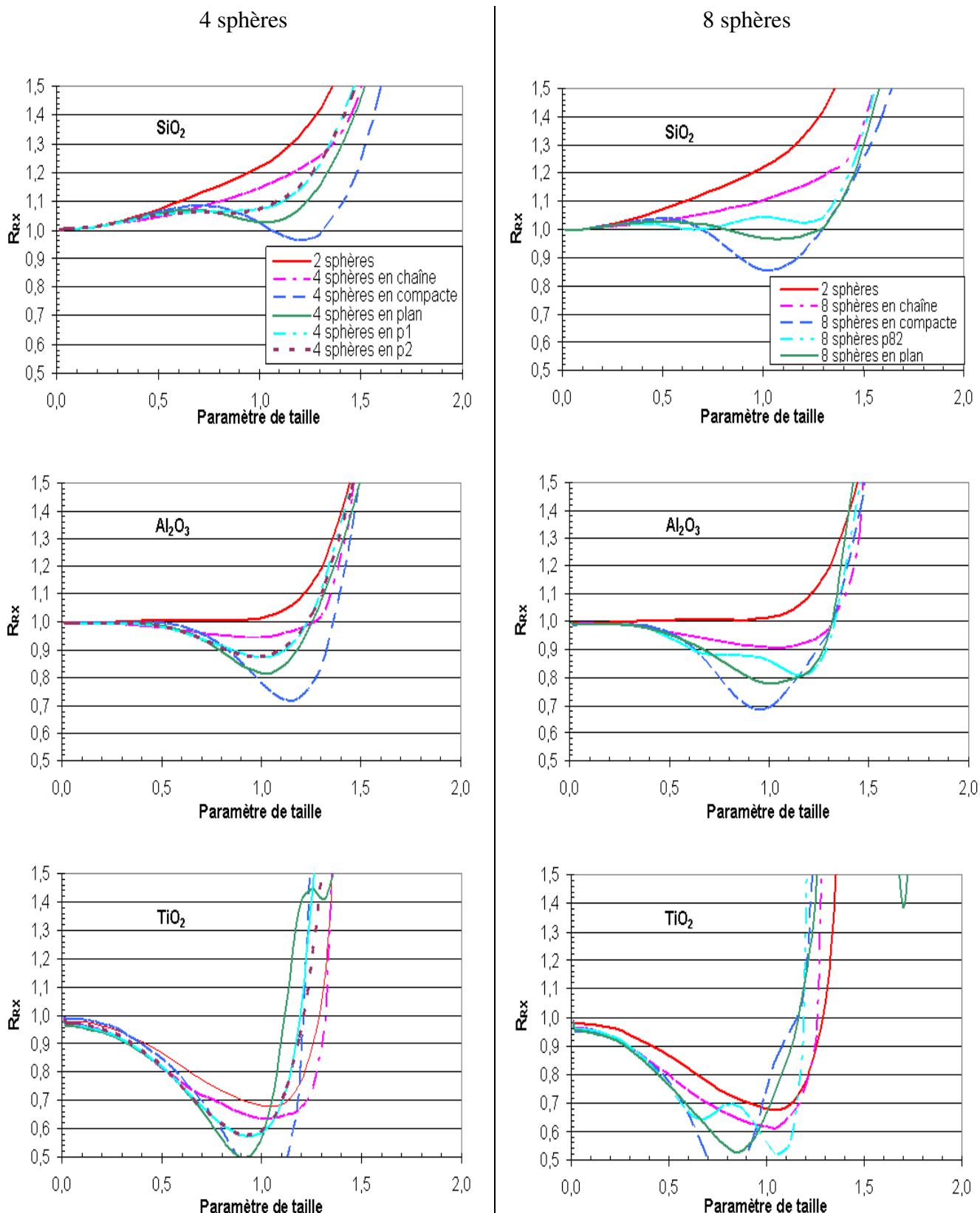
Annexe Figure 10: Domaine de validité de l'approximation de Rayleigh pour des agrégats de 4 et 8 sphères pour les 3 matériaux.
