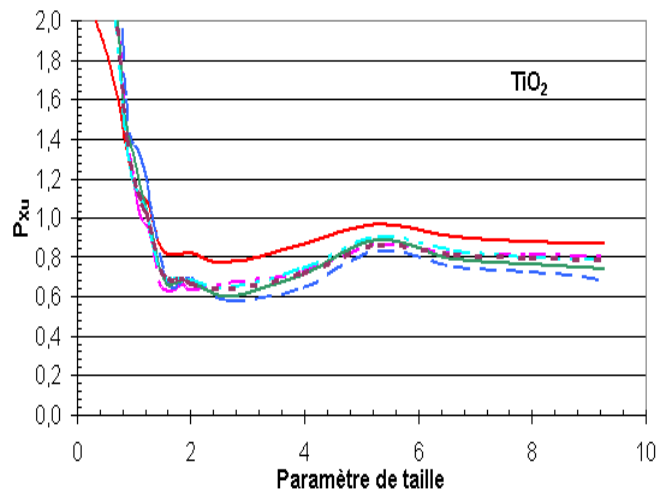
Figure B- III-12: Variation de la section efficace de pression de radiation en fonction de la configuration pour un agrégat composé de 4 sphères primaires.
