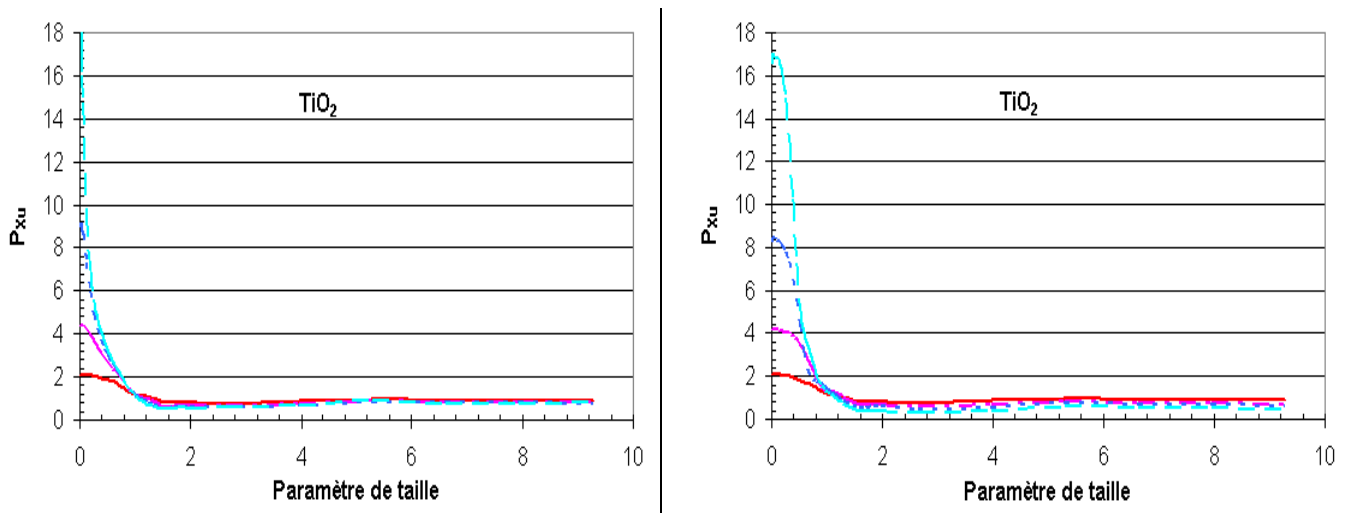
Figure B- III-11: Allure générale des courbes de C_{pr} pour une configuration en chaîne (colonne de gauche) et une configuration compacte (colonne de droite).
