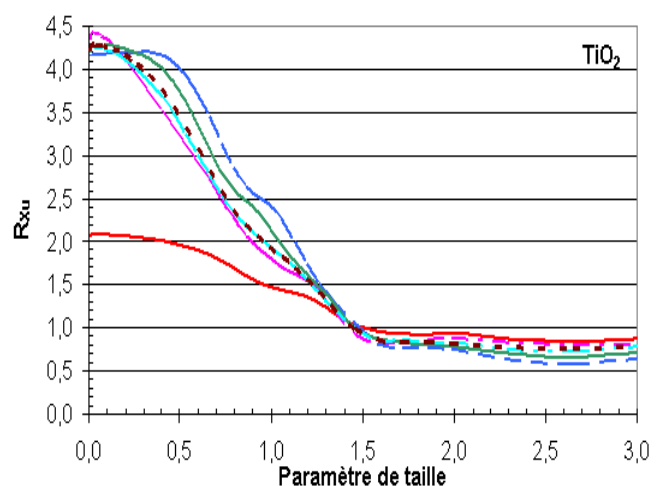
Figure B- III-5: Variation de la section efficace de diffusion en fonction de la configuration pour un agrégat composé de 4 sphères primaires.
