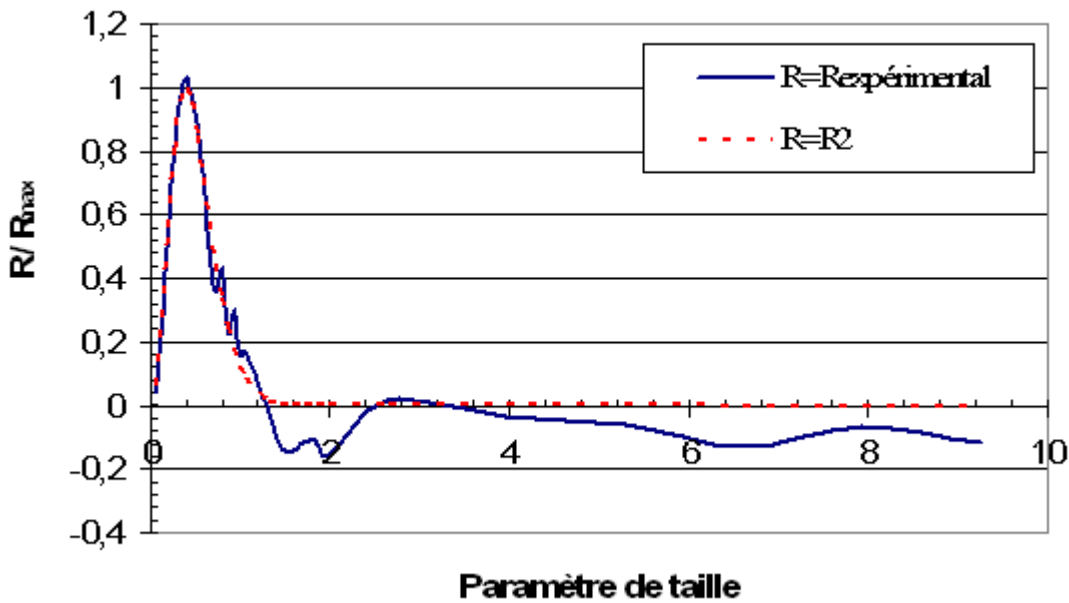
Figure B- VI-3: Concordance de R_2(\alpha)/R_{\max} et R_{\text{expérimental}}(\alpha)/R_{\max} pour un agrégat en configuration en chaîne composé de 8 particules primaires dans le cas de \text{Al}_2\text{O}_3
