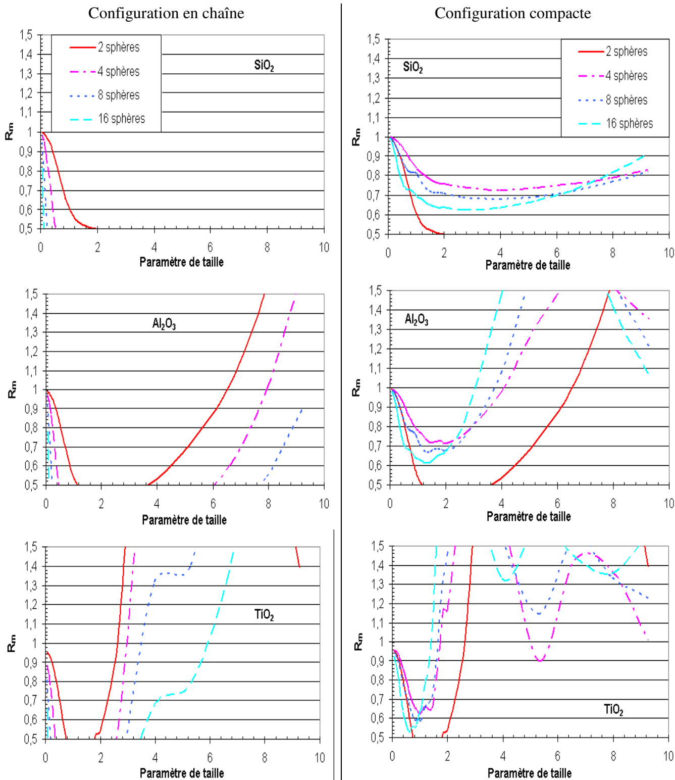
Annexe Figure 18: Méthode de la sphère creuse : Avec R_m \in [0.5, 1.5] en fonction du paramètre de taille, pour les 3 matériaux ( \text{SiO}_2 , \text{Al}_2\text{O}_3 , \text{TiO}_2 ) et suivant 2 configurations : en chaîne (1 ière colonne) et compacte (2 ième colonne).
