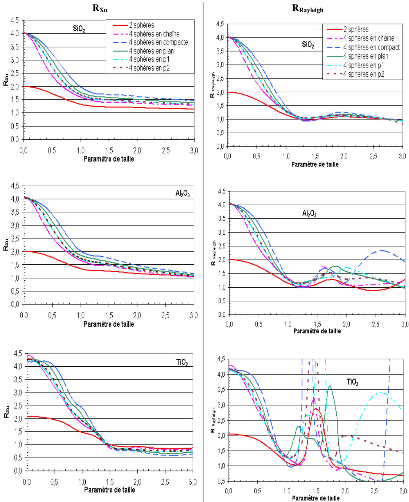
Figure B- IV-1: R_{\text{Rayleigh}} pour les différentes configurations avec 4 sphères suivant le paramètre de taille et les 3 indices ( \text{SiO}_2 , \text{Al}_2\text{O}_3 , \text{TiO}_2 )
