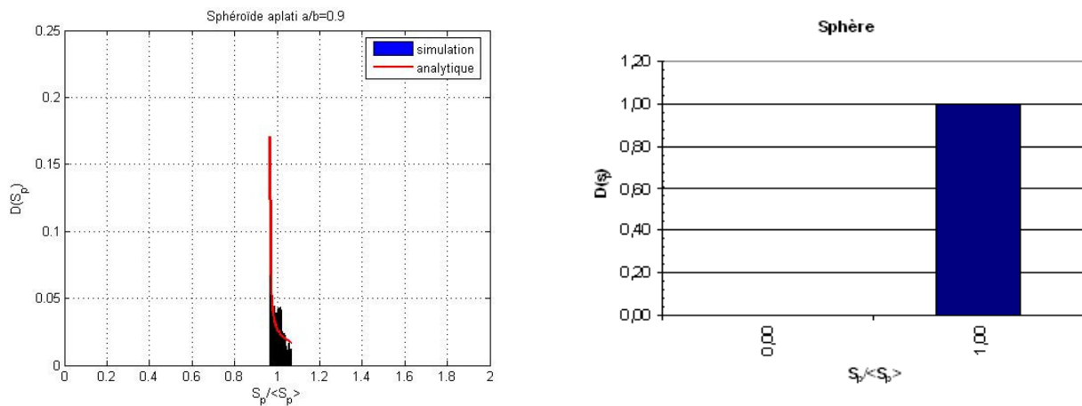
Figure B- I-8: Distribution des surfaces projetées S_p / \langle S_p \rangle normalisées pour un sphéroïde de type aplati
