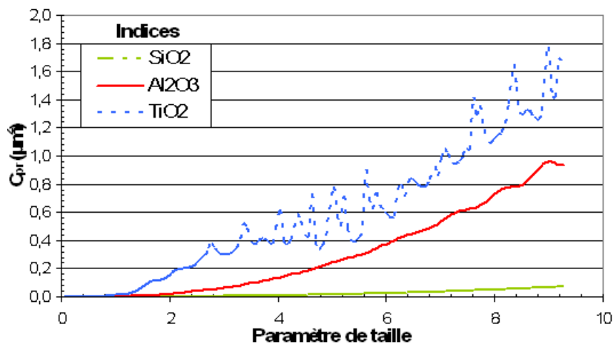
Figure B- III-9: Section efficace de pression de radiation pour les trois matériaux en fonction du paramètre de taille.
