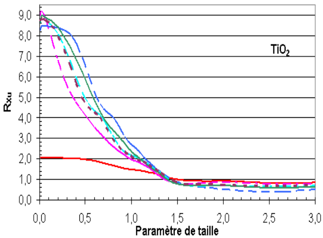
Figure B- III-6: Variation de la section efficace de diffusion en fonction de la configuration pour un agrégat composé de 8 particules primaires.
