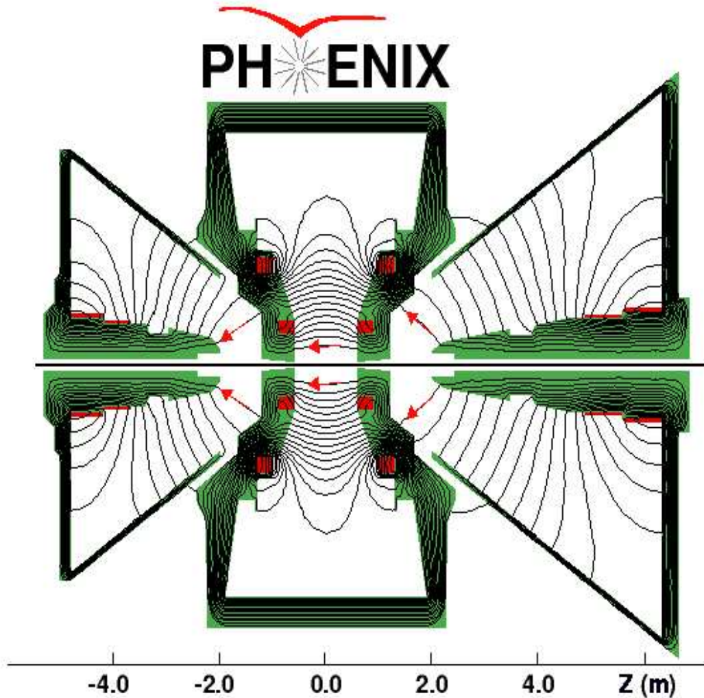
FIG. 2.8 – Carte des champs magnétiques délivrés par les aimants PHENIX.
