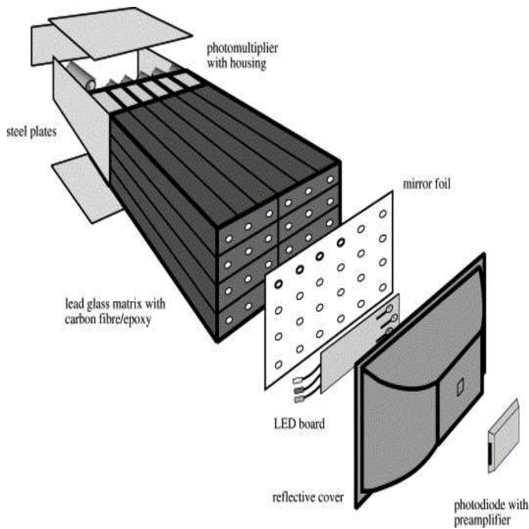
FIG. 2.25 – module PbG1.
