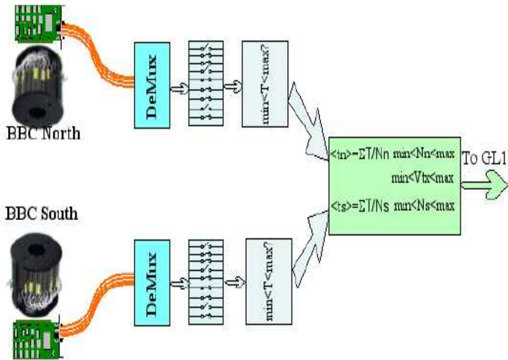
FIG. 2.29 – Mode opératoire d'acquisition de différents paramètres du système Local Level-1.
