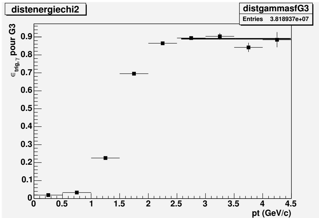
FIG. 4.24 – Efficacité du déclenchement G3 pour les photons.
