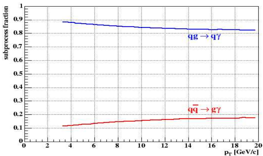
FIG. 1.19 – Fraction des processus gq \rightarrow q\gamma et q\bar{q} \rightarrow g\gamma dans les collisions p+p à \sqrt{s} = 200 GeV en fonction de p_T [61].
