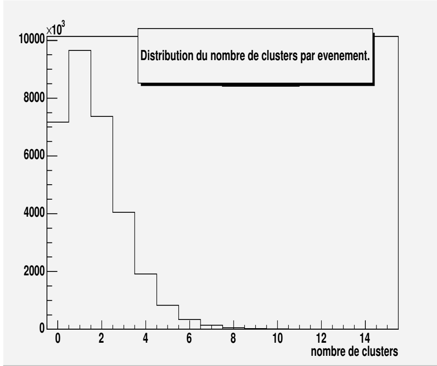
FIG. 3.6 – Distribution du nombre d'agrégats par événement.
