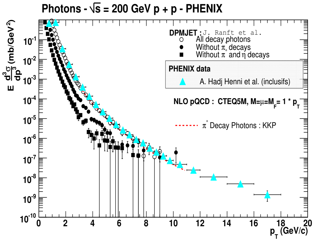
FIG. 6.2 – Spectre des photons inclusifs analysés dans notre travail (triangles pleins), pour les collisions p + p à \sqrt{s} = 200 GeV. Sont également présentés : les résultats de PHOJET/DPMJET concernant les photons issus de la décroissance des divers mésons; les résultats déduits, à l’aide de l’équation (6.6), du spectre de production des pions \pi^0 , calculé par pQCD à l’ordre sous-dominant. Les valeurs concernant les calculs théoriques sont tirées de la figure correspondante dans la référence [84].
