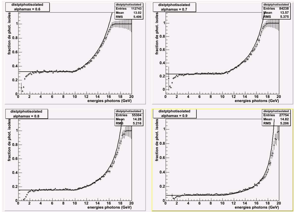
FIG. 3.4 – Fraction de photons isolés pour différentes valeurs \alpha_{\max} dans le cas d'un spectre initial uniforme de \pi^0 . Les lignes continues sont les prédictions équations 3.11 à 3.13.
