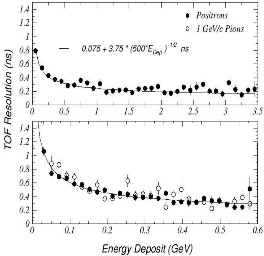
FIG. 2.27 – Résolution en temps de vol des secteurs PbGl en fonction de l'énergie déposée dans un seul module par des positrons d'impulsion 0,5, 0,75, 1,0, 1,5, 2,0, 3,0, et 4,0 GeV/c et pour des pions à 1 GeV/c.
