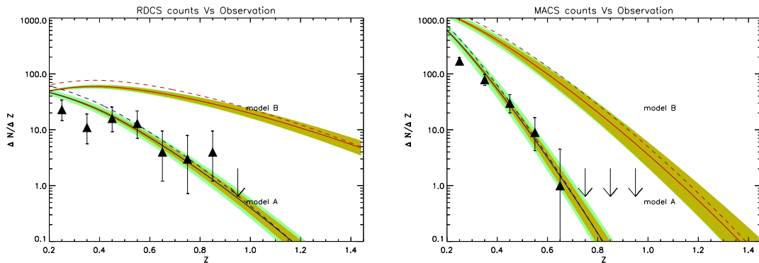
FIG. 5.14 – Effet du choix de la fonction de masse sur les comptages. Illustration dans le cas des deux échantillons “extrêmes” : RDCS et MACS; et pour les fonctions de masse de Press & Schechter (courbes pointillées) et pour celle de Sheth & Tormen (traits pleins).
