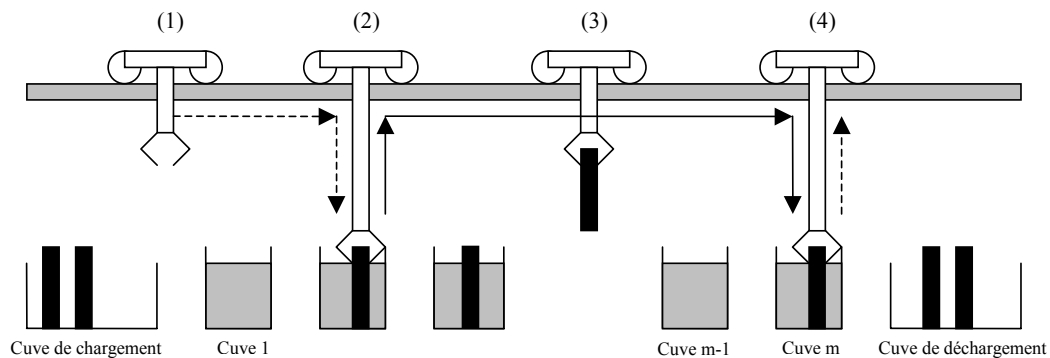
Figure 1.2 – Activités du robot pour le transport d'une pièce
