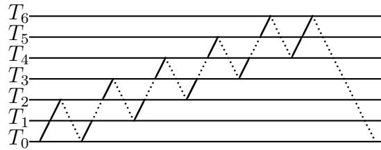
Figure 6.15 – C_1(2) pour m = 5 et p \in [4\delta; 8\delta[
