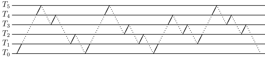
Figure 5.10 – Cycle (043104210321432) optimal pour p \in [10\delta; 12\delta[
