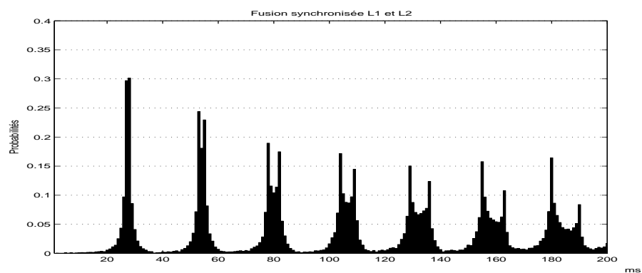
FIG. 3.19 – Distribution empirique : fusion synchronisée (appliquée au GPS)
