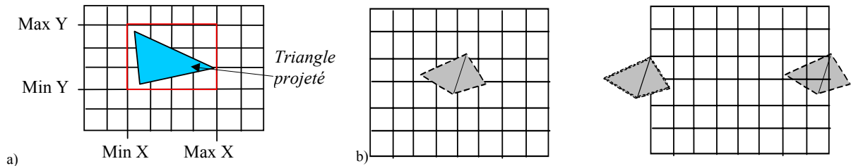
Figure I.15 : a) Bornes d'un triangle projeté sur la couche fictive. b) Projection dans et hors de la maille.
