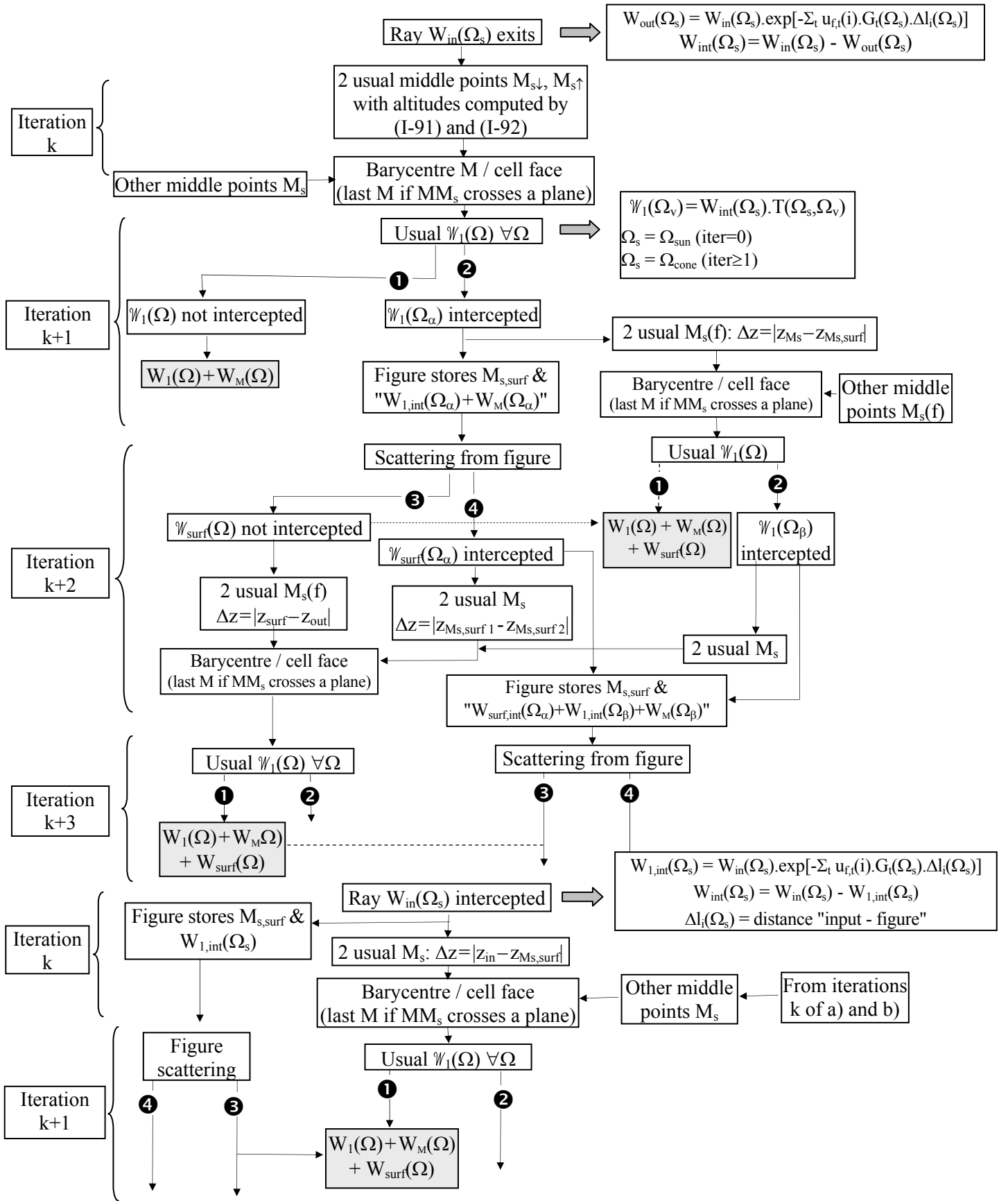
Figure I.32 : Transfert radiatif dans une cellule mixte (turbide + opaque) en mode (R).
