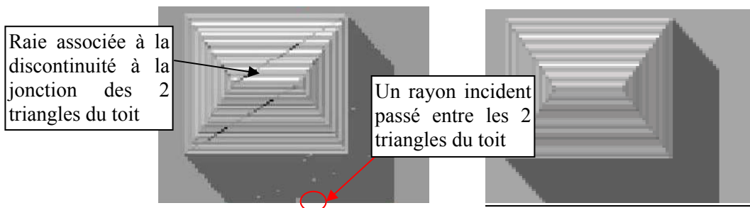
Figure I.25 : Problème du à la réflectance de figures planes coplanaires adjacentes dans une même cellule
