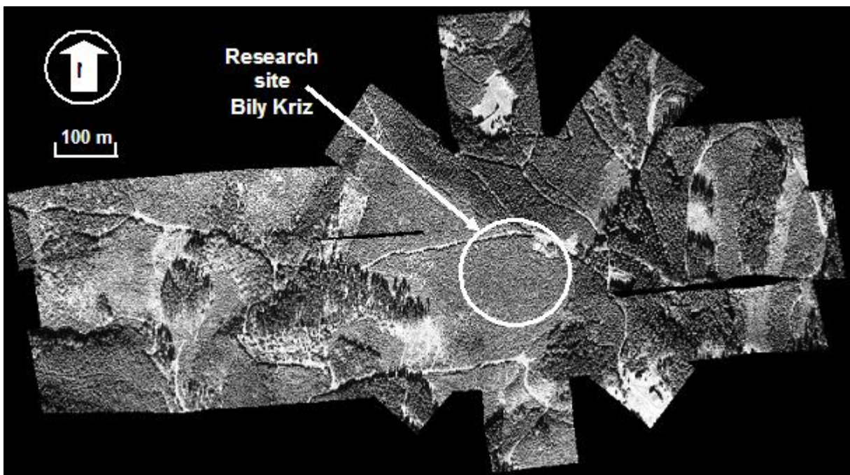
Figure III-8: Six axes de vols ortho-rectifiées du capteur aéroporté AISA Eagle sur le site de Bily Kriz (Monts Beskydy, République Tchèque; 18.54°E, 49.50°N, 936m d'altitude). Résolution spatiale : 40cm.
