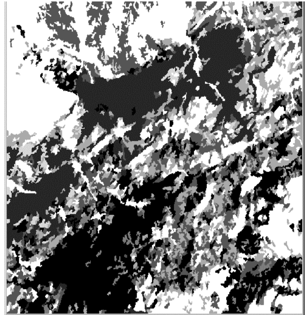
Figure F: Carte d'occupation du sol (Maroc, 48 x 44 km) et simulation DART associée (droite).
