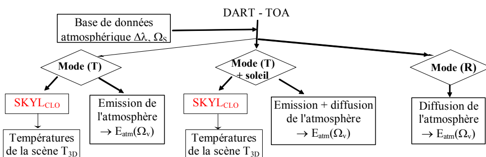
Figure I.52: Produits de {DART monospectral + T.R. atmosphérique. Modes (R) et (T)}.
