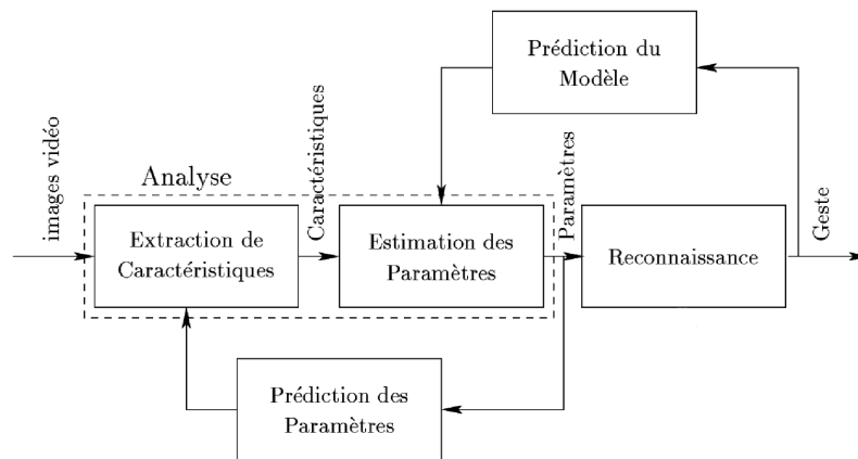
FIG. 5.3 – Synoptique classique d'un système d'analyse/reconnaissance de gestes [Pavlovic et al., 1997]
