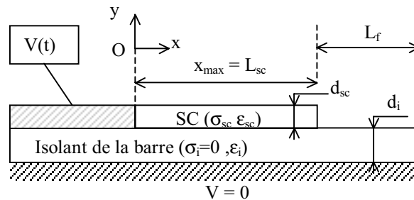
Figure 10 : Schématisation 2D d'une couche mince de SC appliquée sur un isolant parfait.
