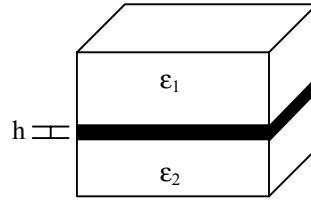
Figure 24 : Région conductrice d'épaisseur h assez fine, comprise entre deux régions diélectriques de permittivités respectives \varepsilon_1 et \varepsilon_2 .
