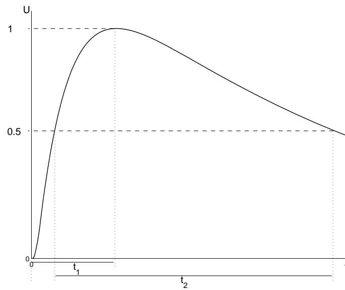
Figure 2 : Relevé des temps caractéristiques sur une onde de choc type manœuvre.
