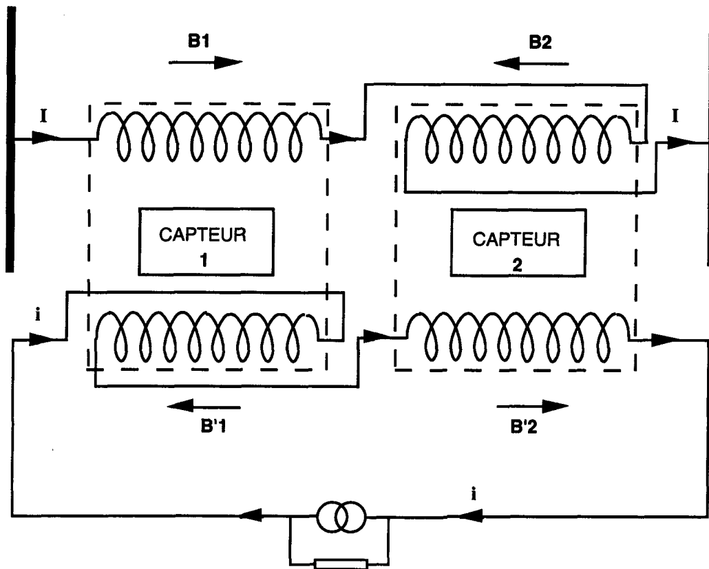
Figure 2.1 - Schéma de principe de l'électromètre
