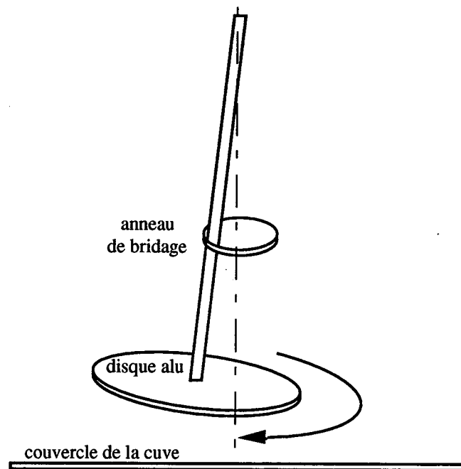
Figure 3.11 - Système de rotation
