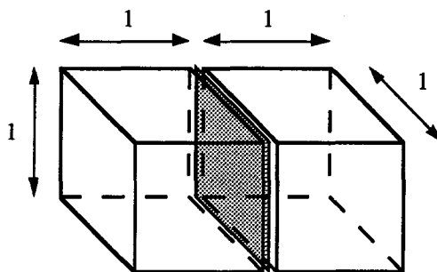
Figure 4.12 - Géométrie test
