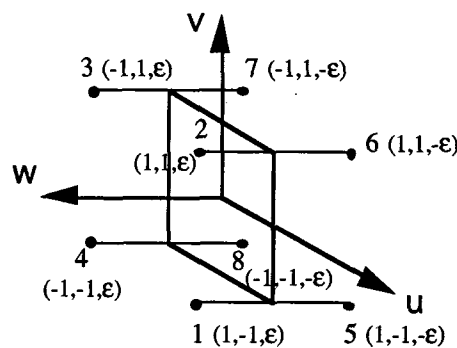
Figure 4.4 - Exemple d'élément interfacial du premier ordre en 3D
