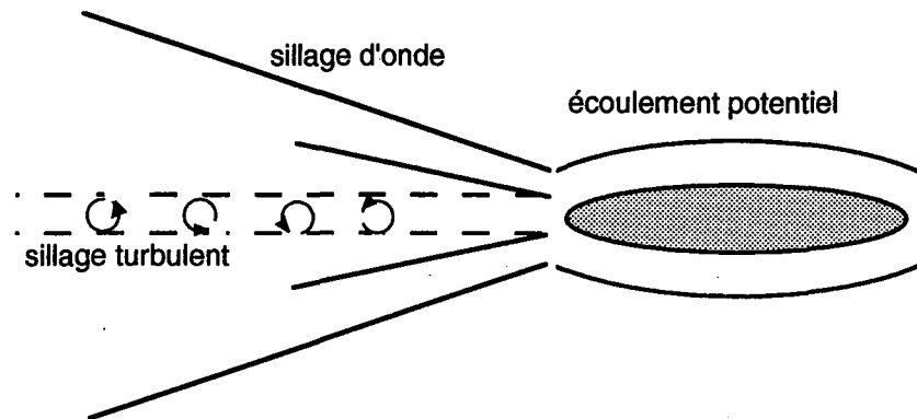
Figure 1.11 - Composantes du sillage d'un bâtiment immergé
