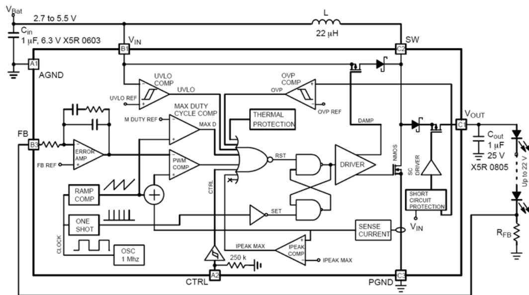
FIG. 3.35 – Schéma synoptique du convertisseur DC/DC
