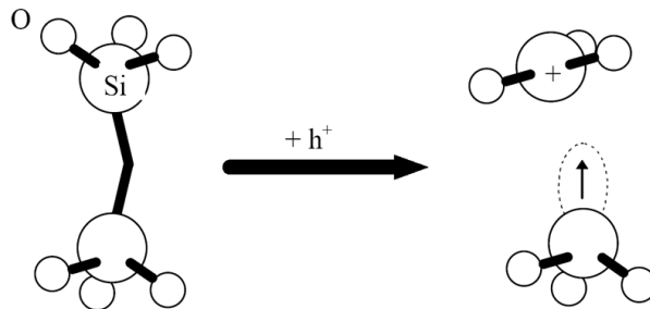
FIG. 1.12 – Création d'un centre E' (piégeage d'un trou)
