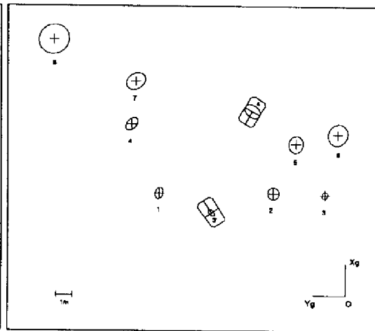
FIG. VII.15 - Le robot effectue un grand déplacement jusqu'à la position 4, l'incertitude de l'estimée de sa position augmente de manière significative.
