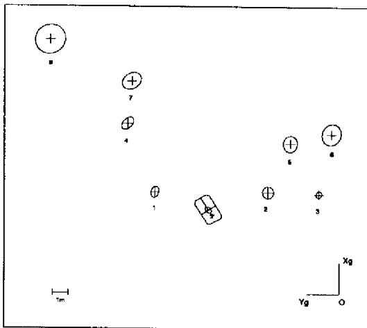
FIG. VII.14 - Carte stochastique à l'issue de la troisième perception. Le robot est recalé (position 3'), les deux sommets des amers revus sont fusionnés et le nouvel amer est ajouté à la carte. On observe à nouveau une diminution des incertitudes du robot et des amers reconnus (cf figure VII.12)
