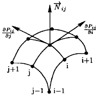
FIG. IV.3 – Principe de l'évaluation des normales
