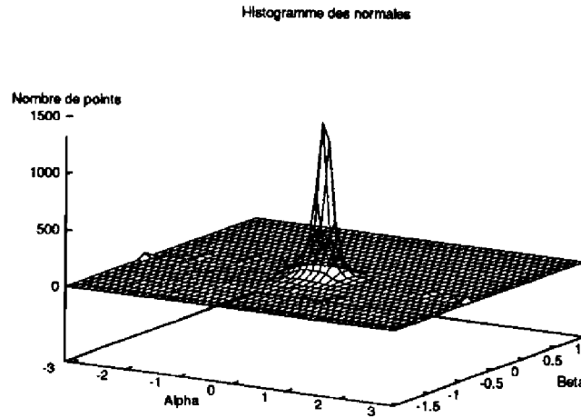
FIG. IV.6 – Histogramme bi-variable H des normales. Le sol étant majoritaire et uniforme, il apparaît comme un pic dans l'histogramme.
